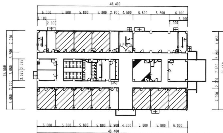
125号建物2階平面図 S=1:600
