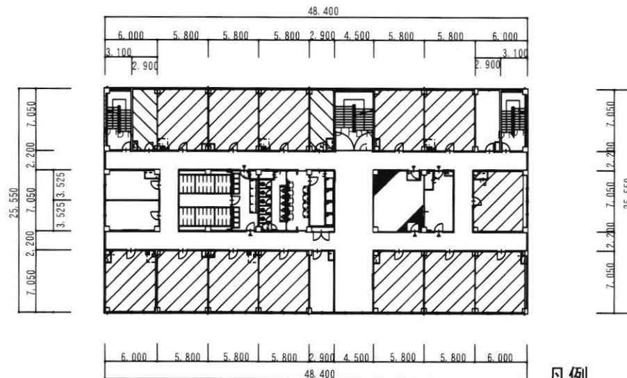
125号建物3階平面図 S=1:600
