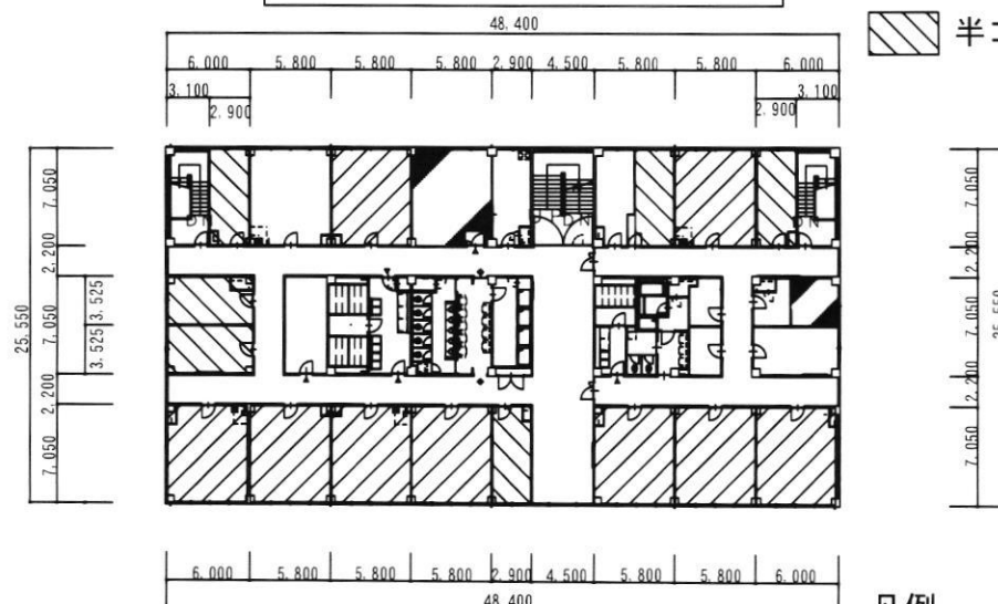
125号建物4階平面図 S=1:600
