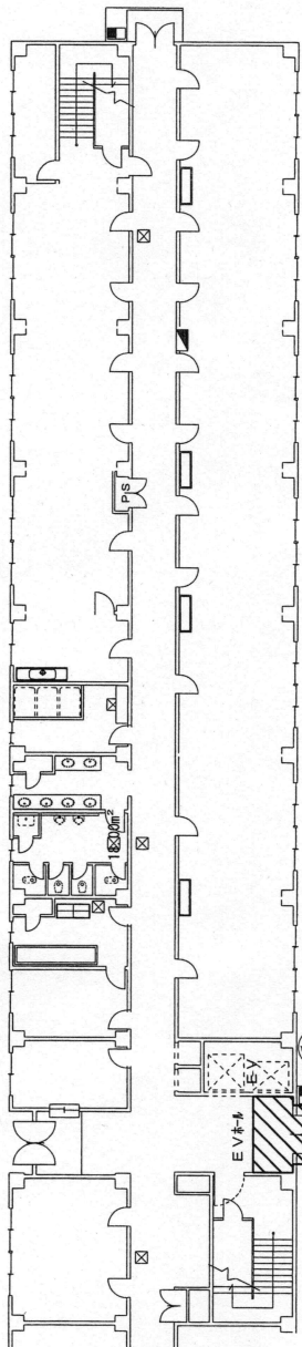
86号建物平面図
