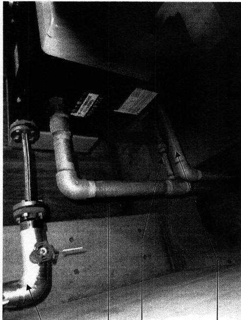
No.100号建物消火ポンプ現況写真②
