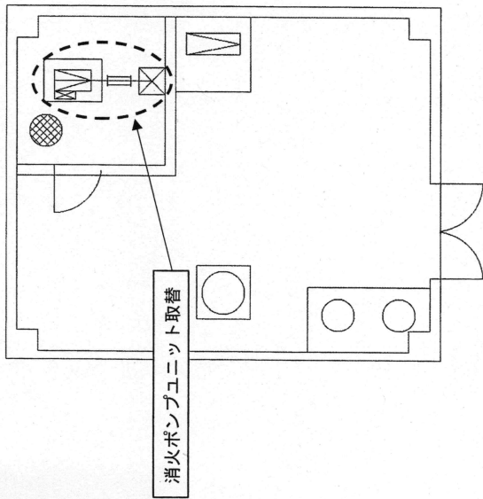
No.100号建物機械室平面図 S=1:X
