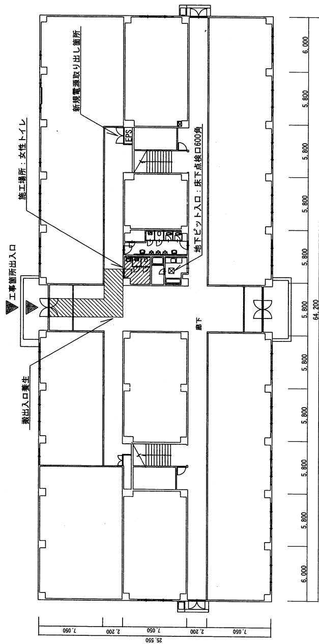
96号建物1階平面図 S=1:300
