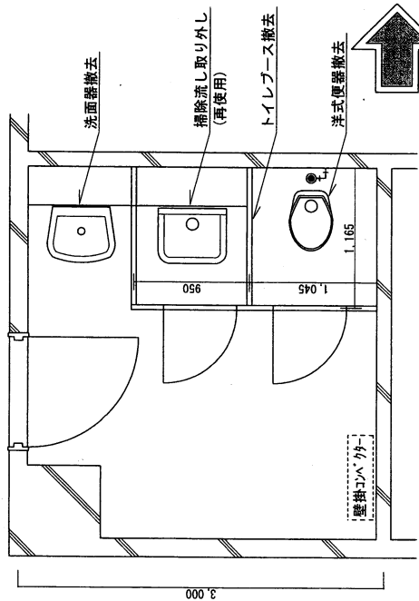
1 F女性トイシ平面図(改修前) S=1:40
