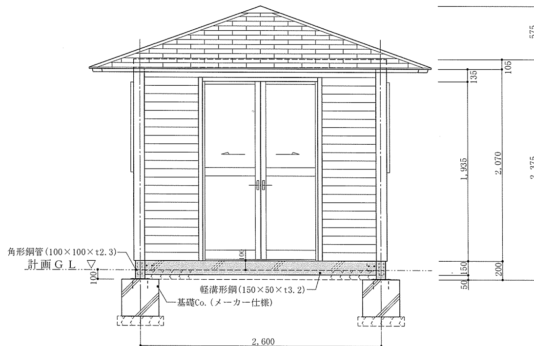
南側立面図 S=1/40
