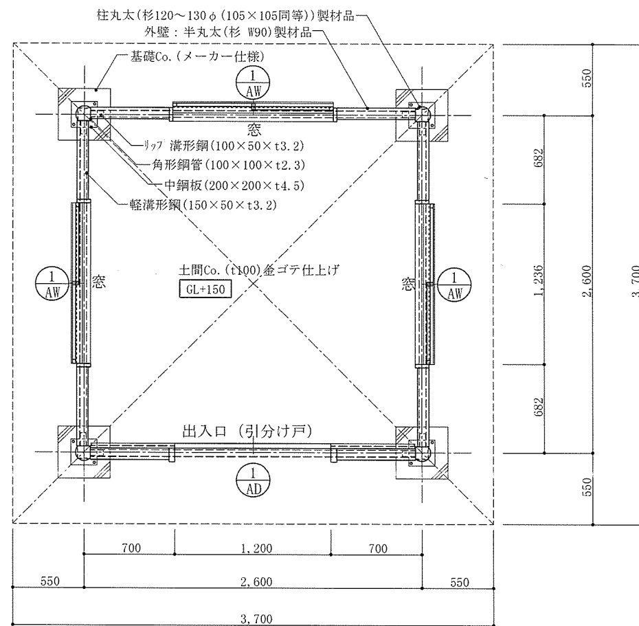
平面図 S=1/40
