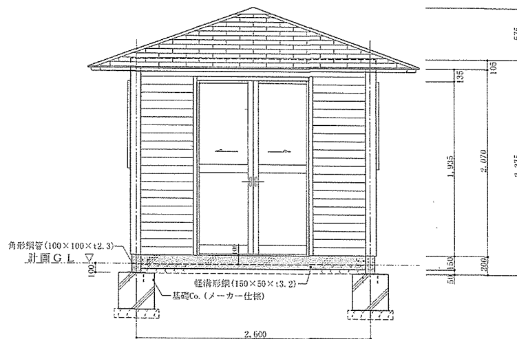
南側立面図 S=1/40
