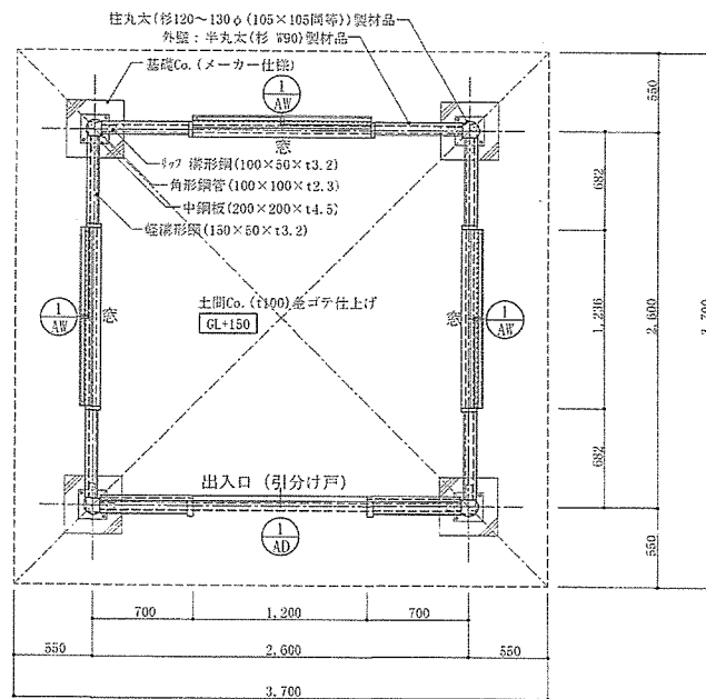
平面図 S=1/40
