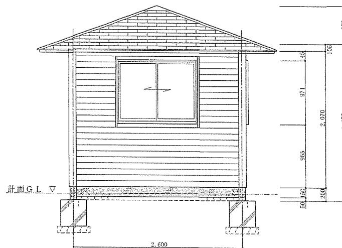
東(北・西)側立面図 S=1/40
