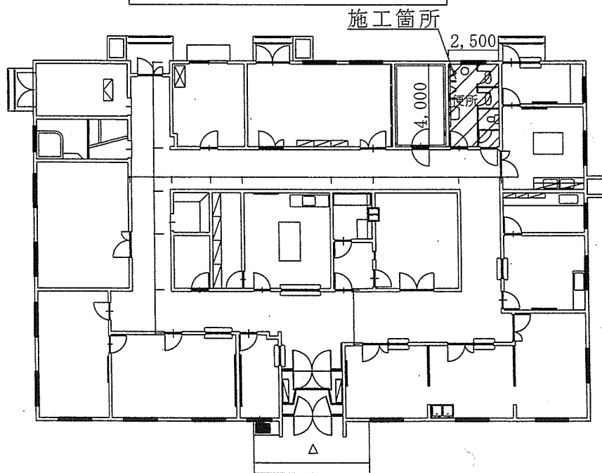
116号建物平面図 1:250
