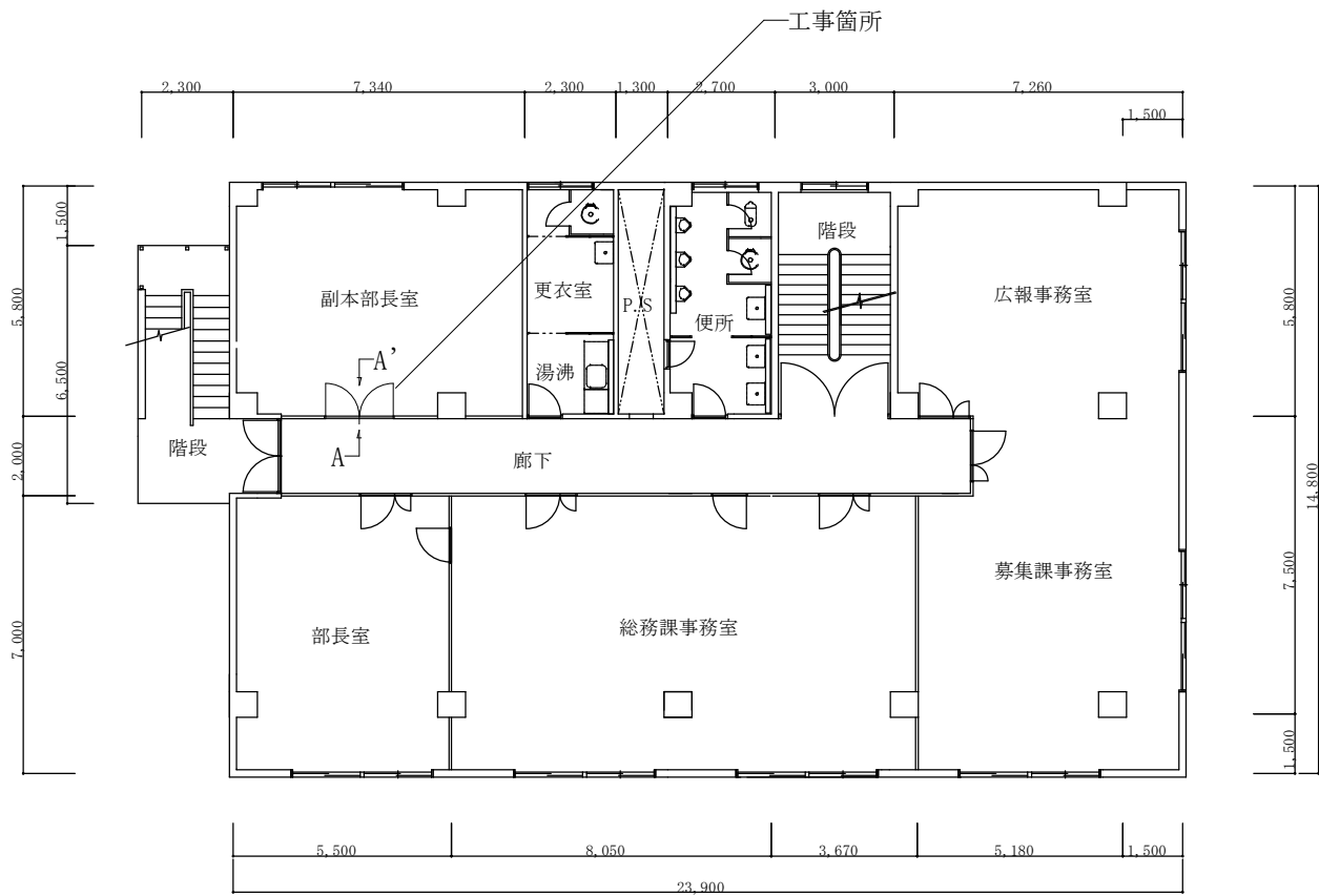
長崎地本庁舎 2階平面図 S=1:200
