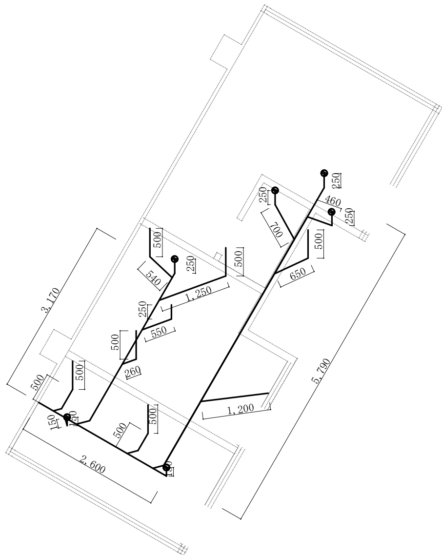
警衛所便所排水管詳細図 S = 1/60
