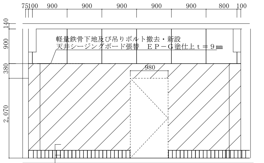
4 2 号建物 2 階男子便所展開 A 面 1 : 6 0
