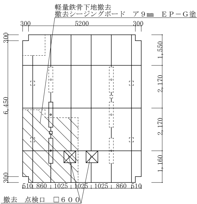
改修前 4 2 号建物 1 階女子便所天井伏図 1 : 8 0
