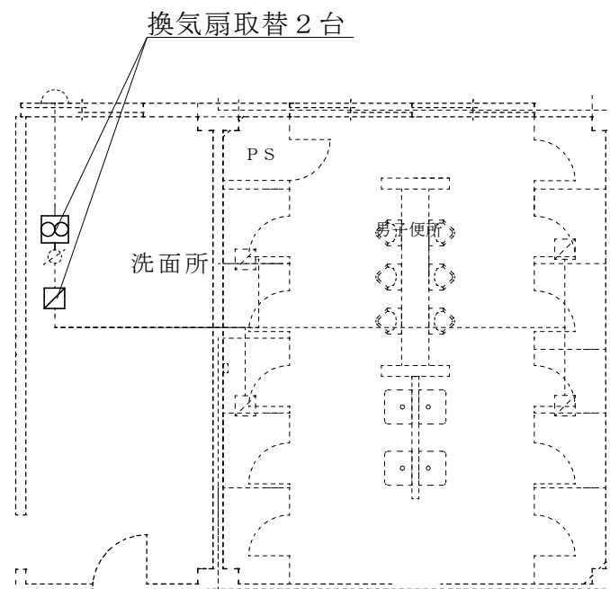
4 2 号建物 2 階洗面所・便所換気設備平面図
