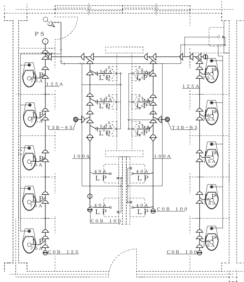
2階床下排水平面図 1 : 6 0
