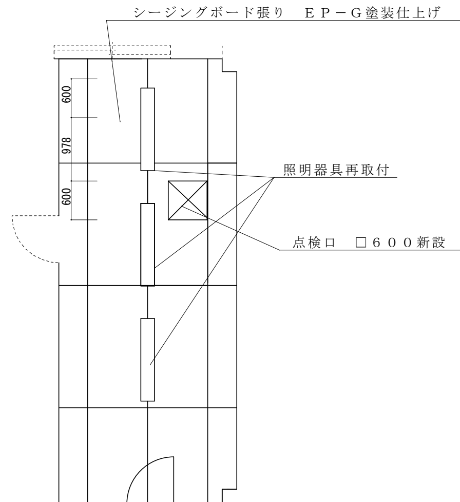
改修後 4 2 号建物 2 階洗面所天井伏図 1 : 5 0
