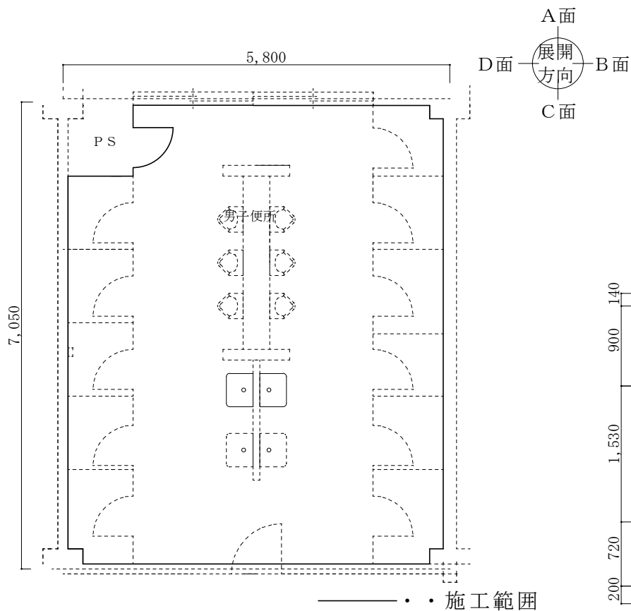
4 2 号建物 2 階便所平面図 1 : 1 0 0
