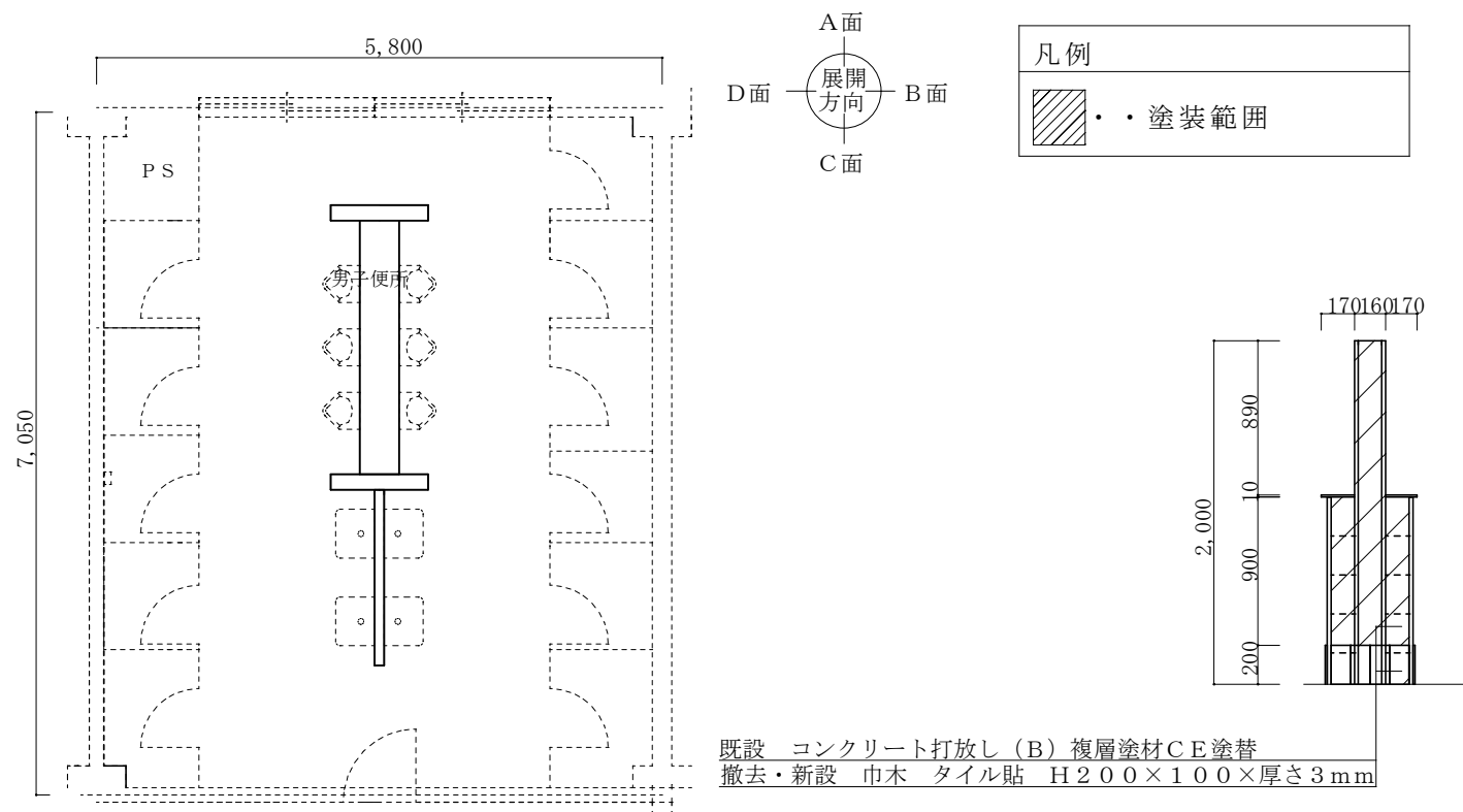
2階便所カランバック展開図A面 1 : 4 0
