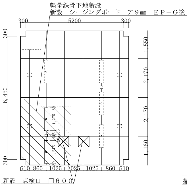
改修後 4 2 号建物 1 階女子便所天井伏図 1 : 8 0
