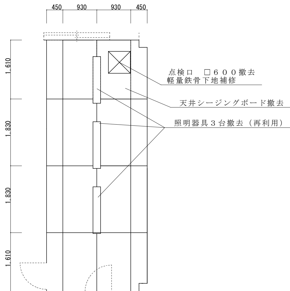
改修前 4 2 号建物 2 階洗面所天井伏図 1 : 5 0
