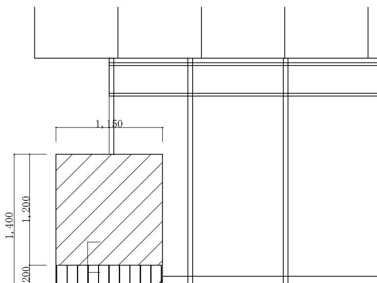
1階便所カランバック展開図A面 1 : 4 0
