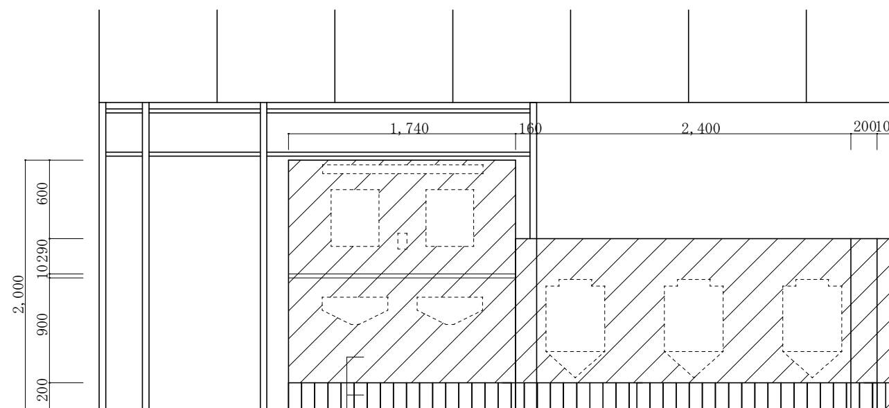
1階便所カランバック展開図B面 1 : 4 0
