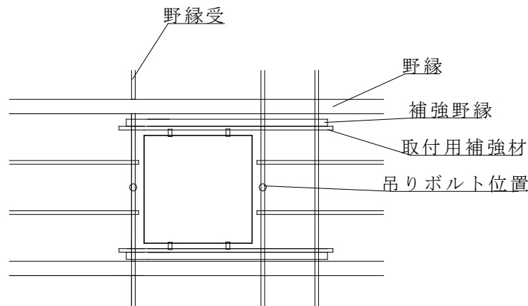
点検口補強標準図 1 : 5 0
