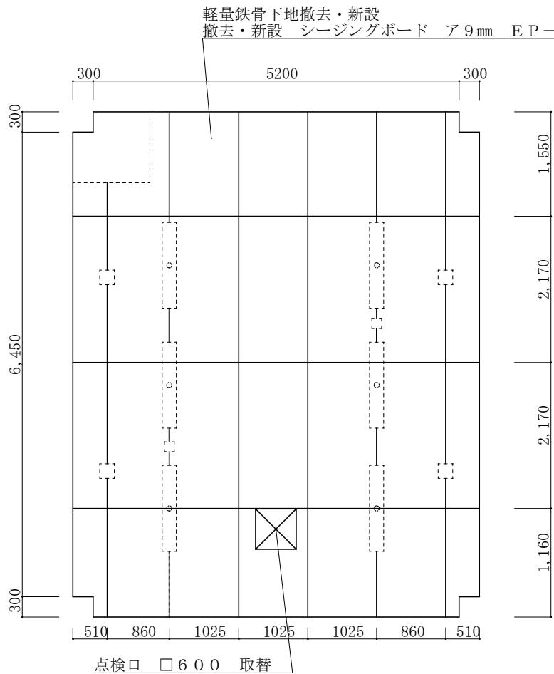
4 2 号建物 2 階便所平面図 1 : 1 0 0
