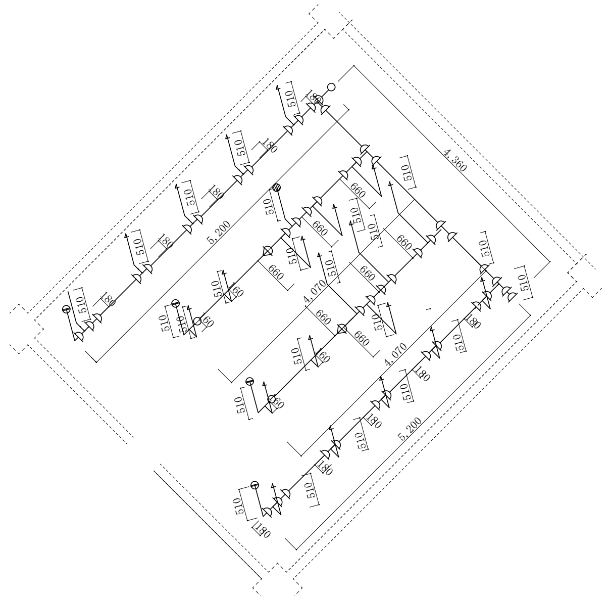
既設排水管詳細図 1 : 6 0
