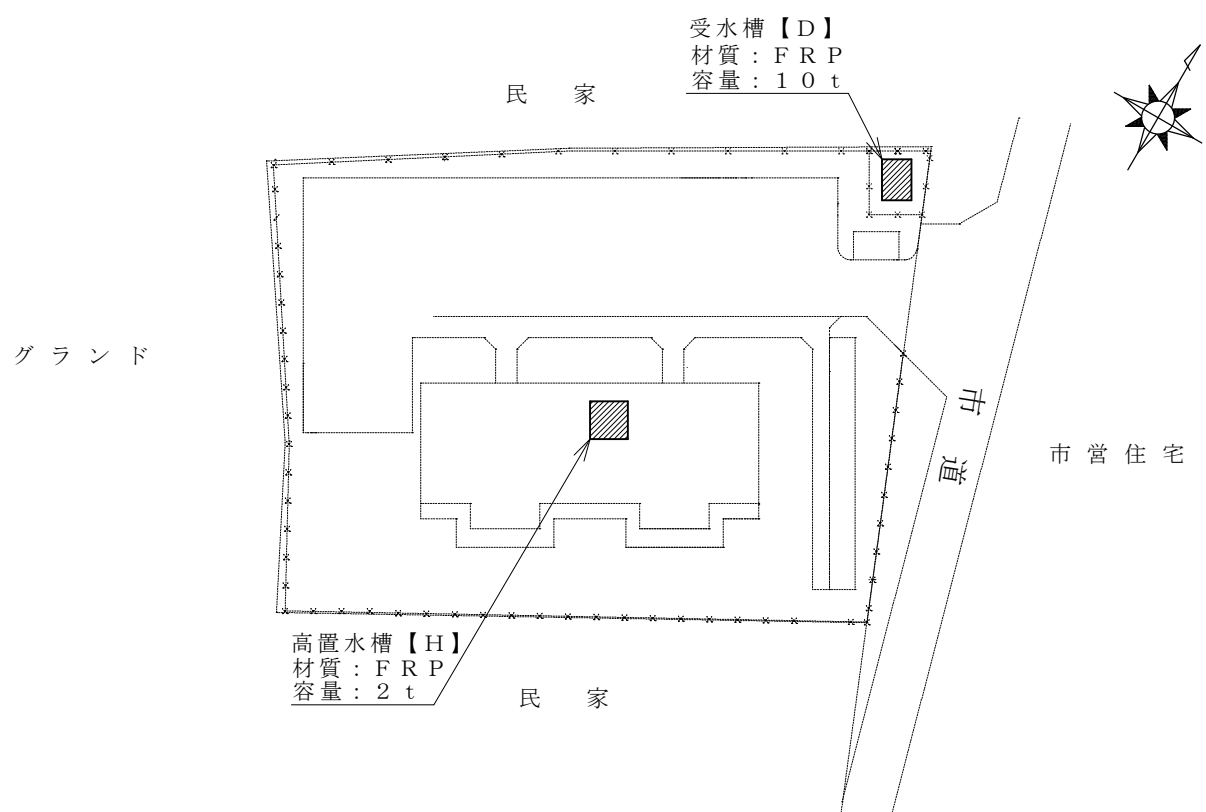
第一小路口宿舎C棟配置図
