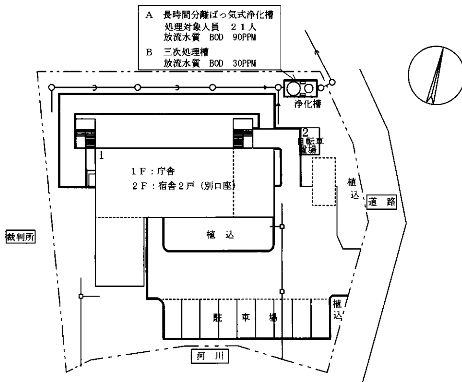
配置図 1/500
