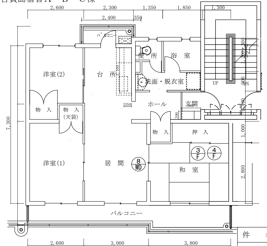
古賀島宿舎 A・B・C 棟平面図 1/100
