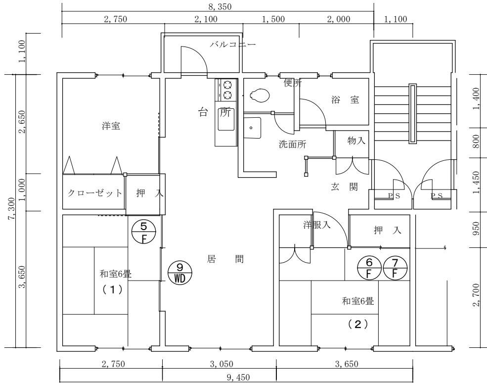
第二小路口宿舎 A 棟・B 棟平面図 1/100
