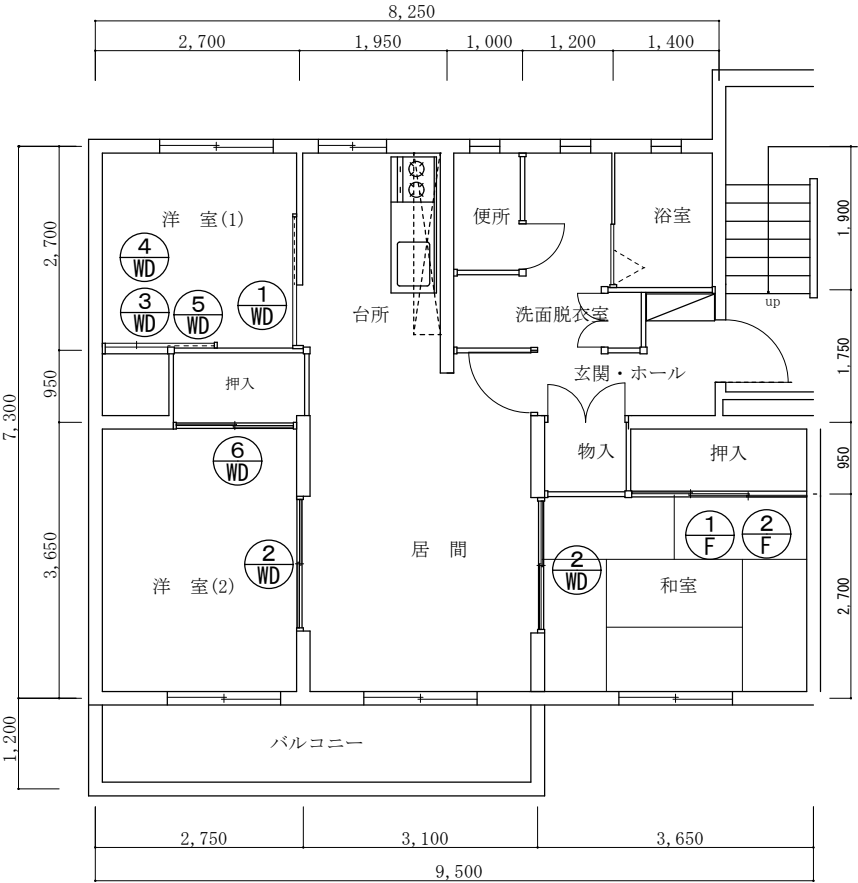
森園宿舎 6 棟 7 棟 C 規格平面図 1/100
