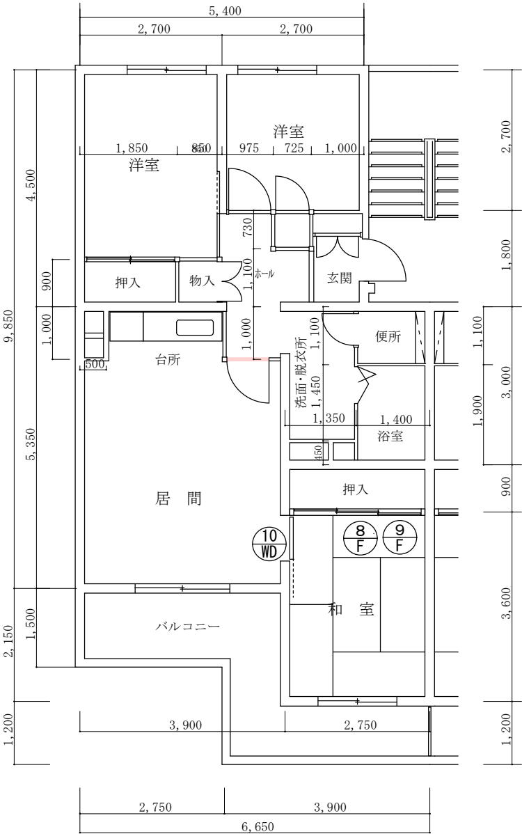
第一小路口宿舎 C 棟平面図 1/100
