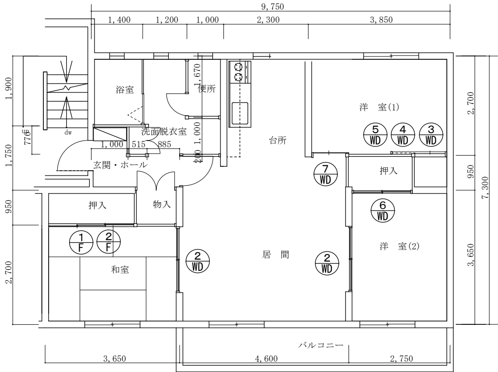
森園宿舎 7 棟 D 規格平面図 1/100
