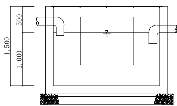
No.10油分離槽 S=1:70
