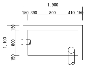
No.10油分離槽 S=1:70
