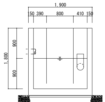
No.12油分離槽 S=1:70
