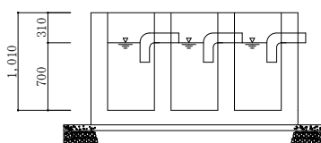
No.8油分離槽 S=1:70
