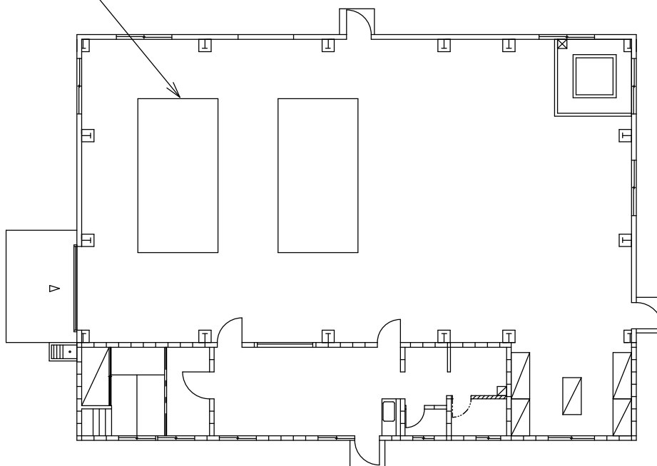
ボイラー室平面図 S=NON SCALE
