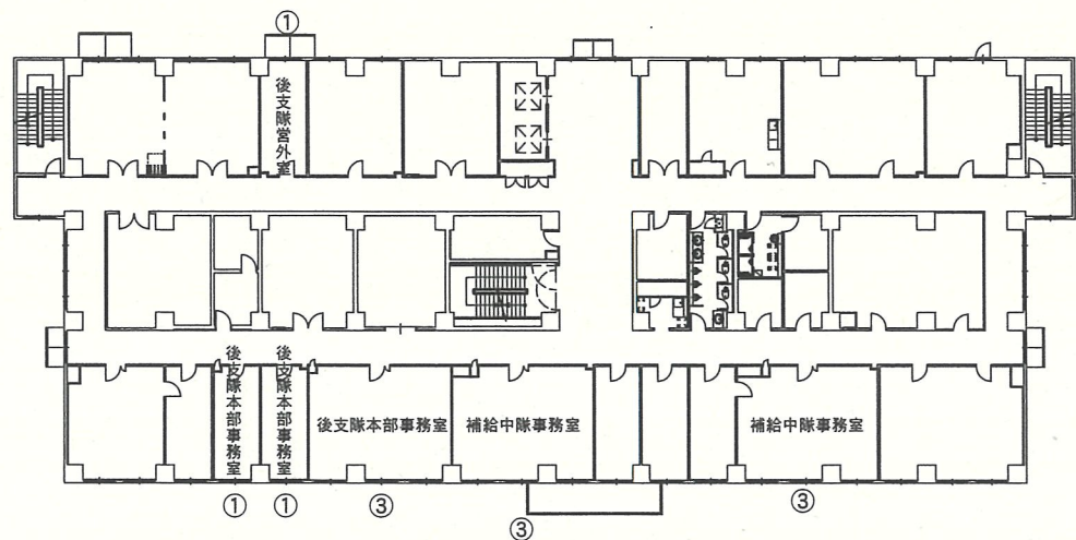
151号隊舎2階平面図
