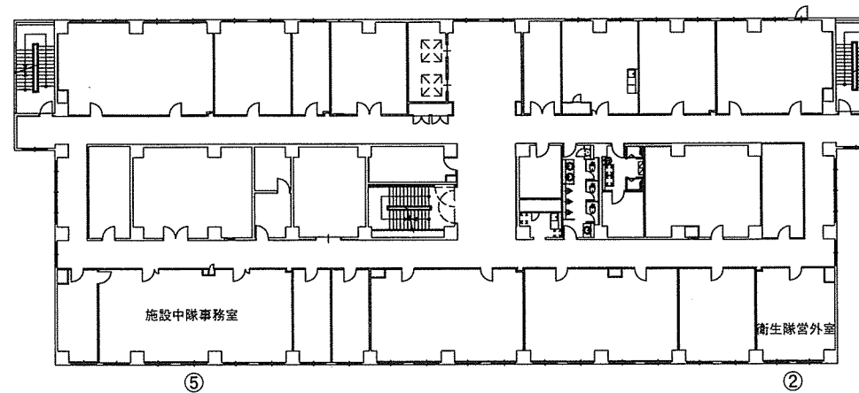
151号隊舎4階平面図
