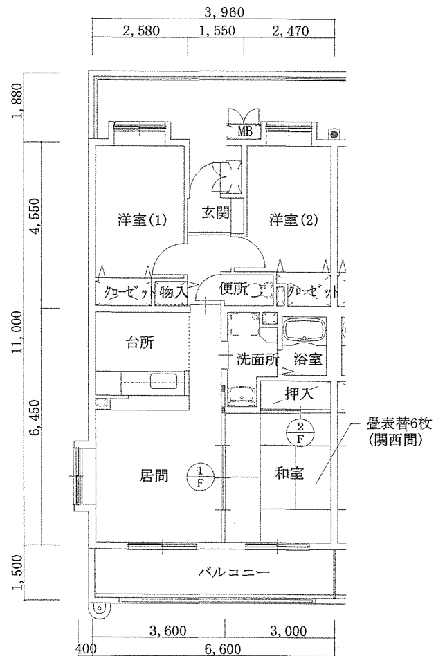
宿舍平面図 S=1/100
