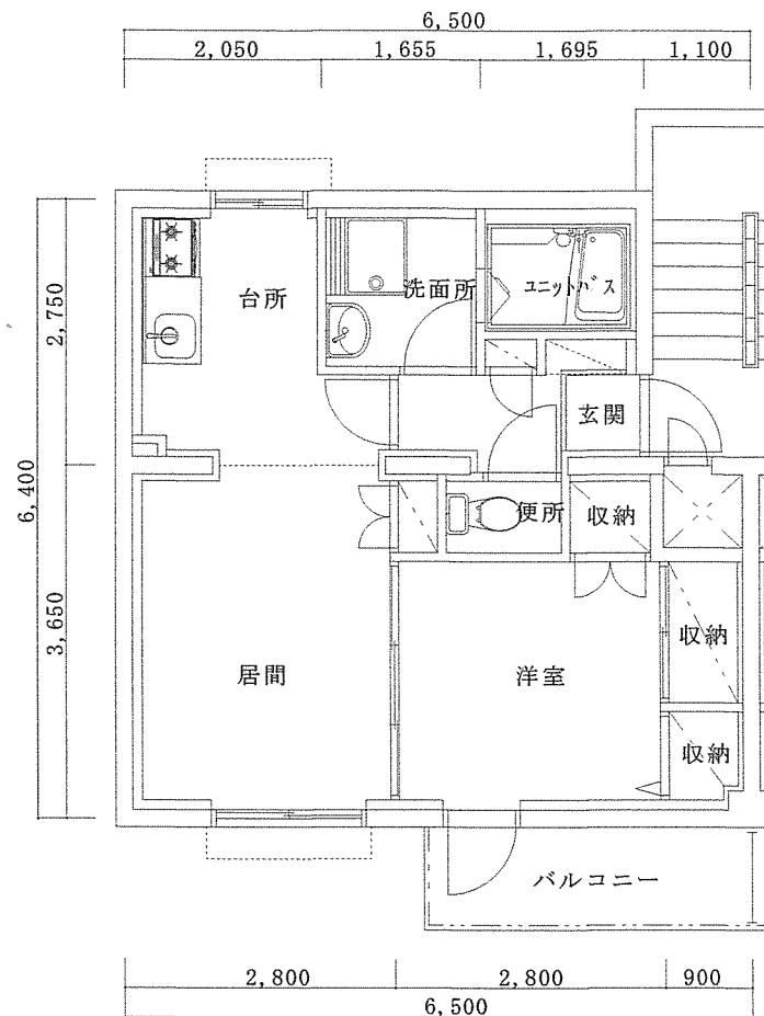
宿舎平面図 S=1/60
