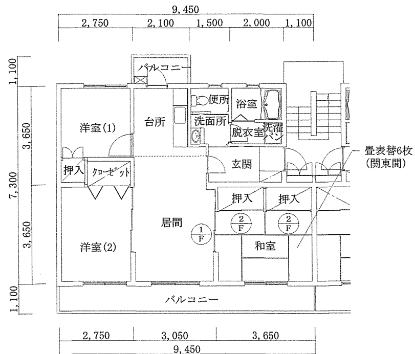
宿舎平面図 S=1/100
