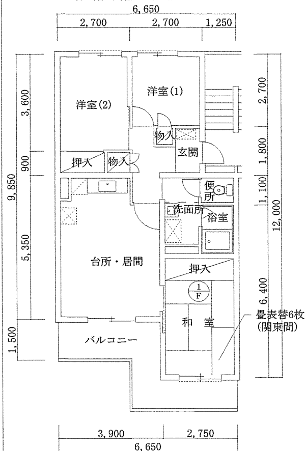
宿舍平面図 (3LKタイプ) S=1/100
