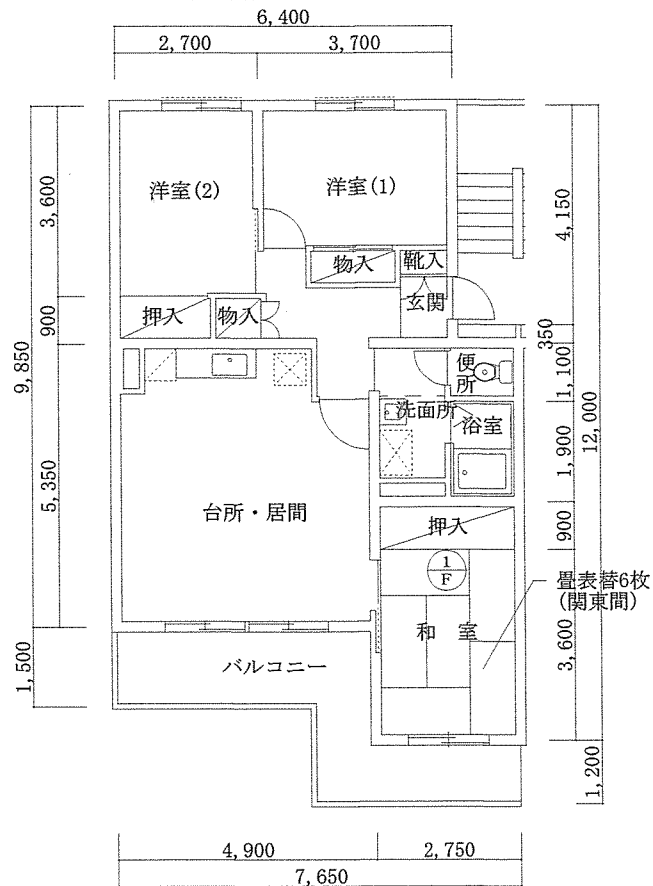
宿舍平面図 (3LDKタイプ) S=1/100
