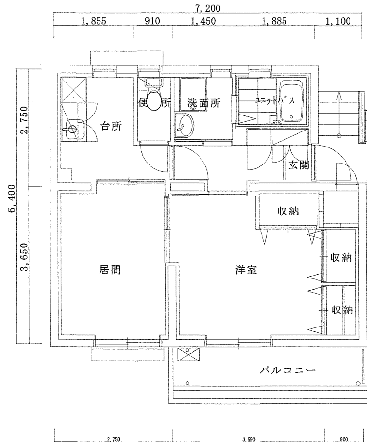
宿舎平面図 S=1/60
