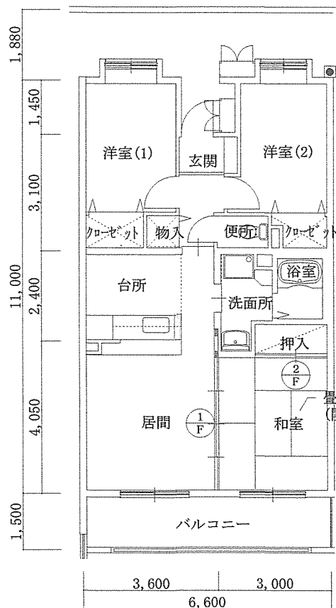
宿舍平面図(3LKタイプ) S=1/100
