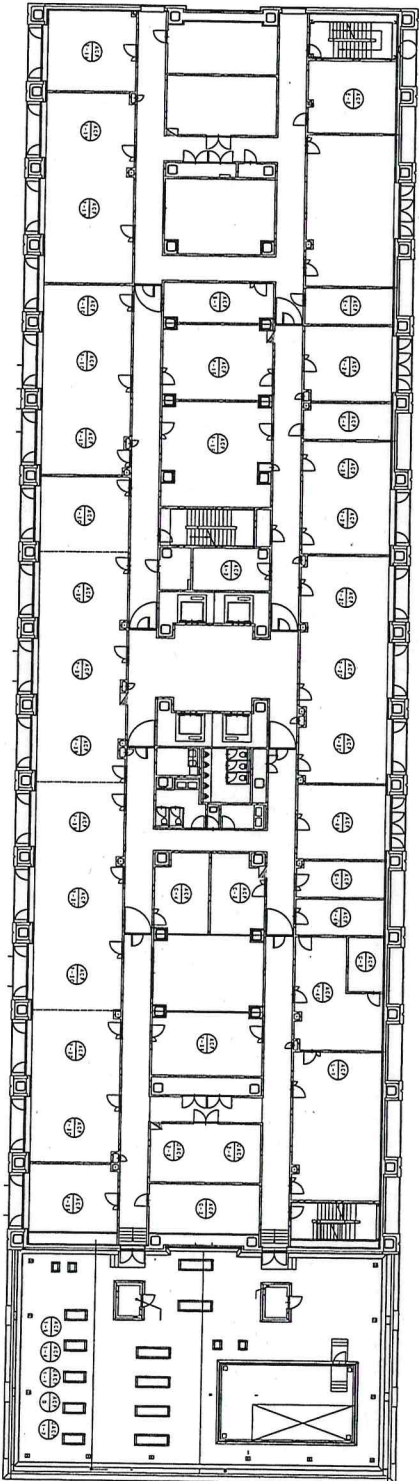
1号建物 2階平面図
