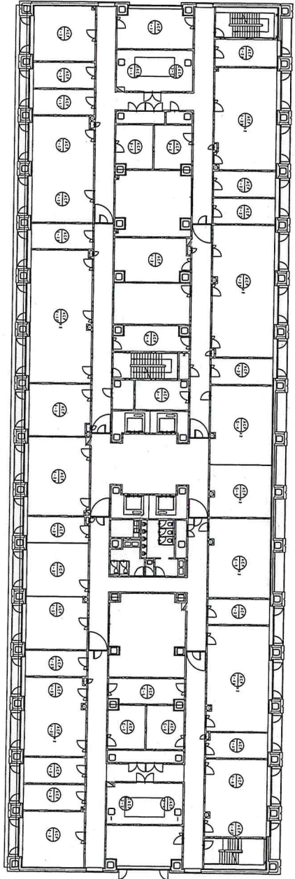
1号建物 3階平面図
