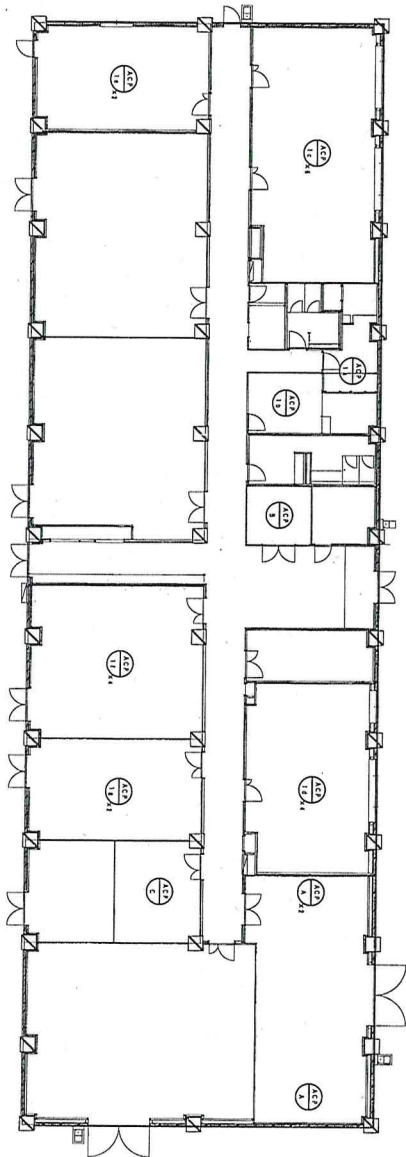
4号建物 1階平面図
