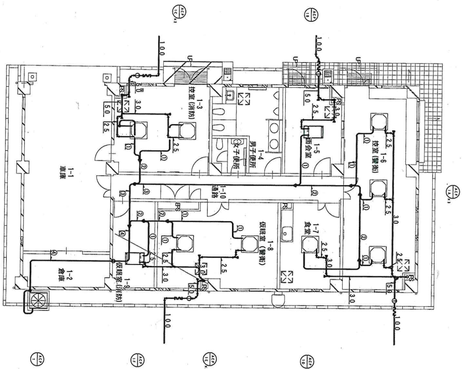
7号建物 平面図 S=1/200
