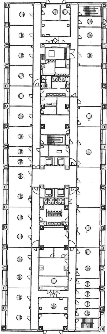
1号建物 5階平面図
