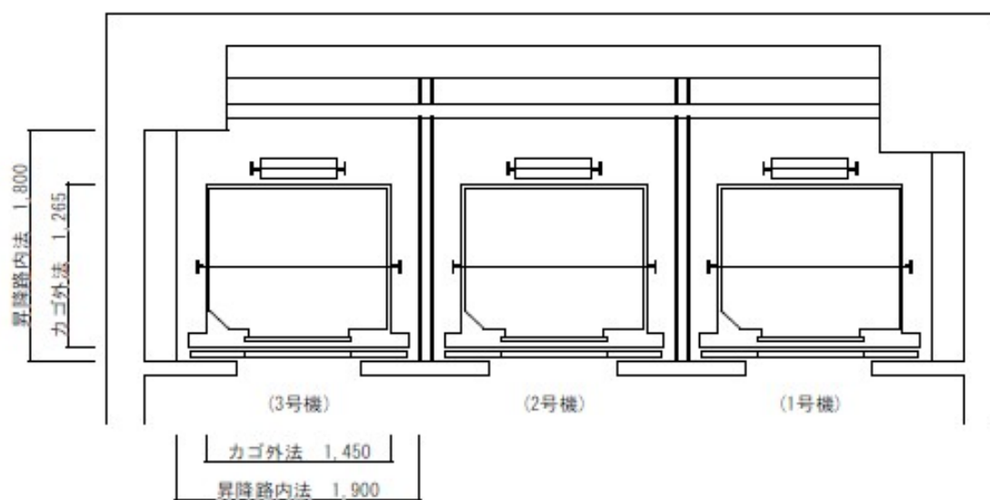
昇降路平面図
