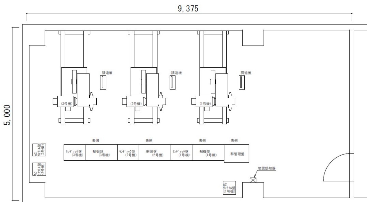
機械室平面図
