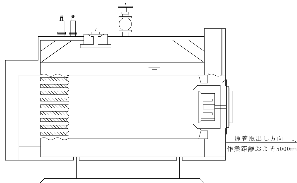
B-B' 断面図
