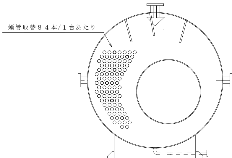
A-A' 断面図
