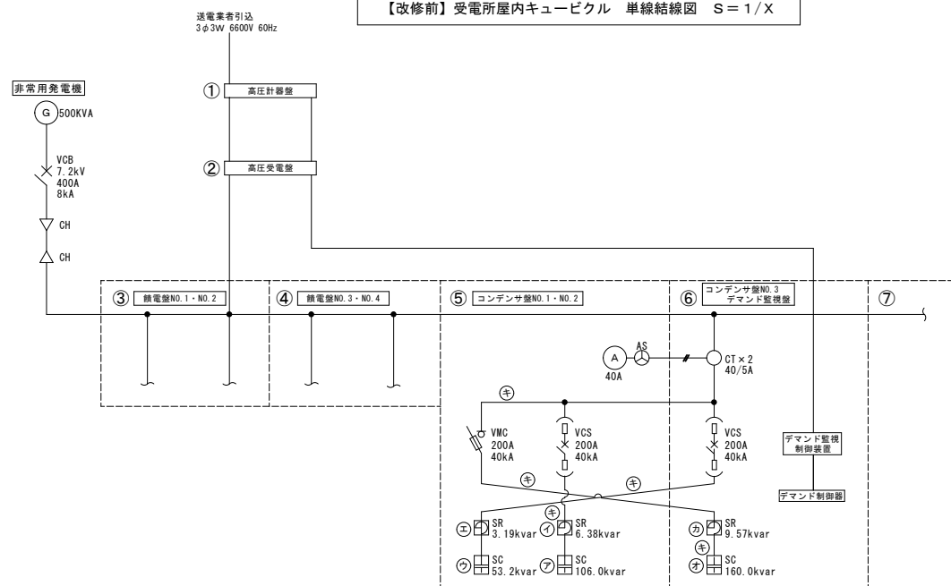
【改修後】受電所屋内キュービクル 単線結線図 S=1/X
