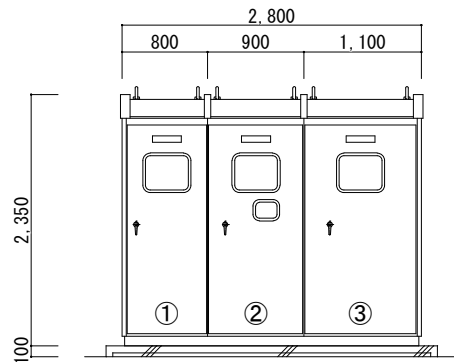
224号屋外キュービクル 正面図 S=1/50
