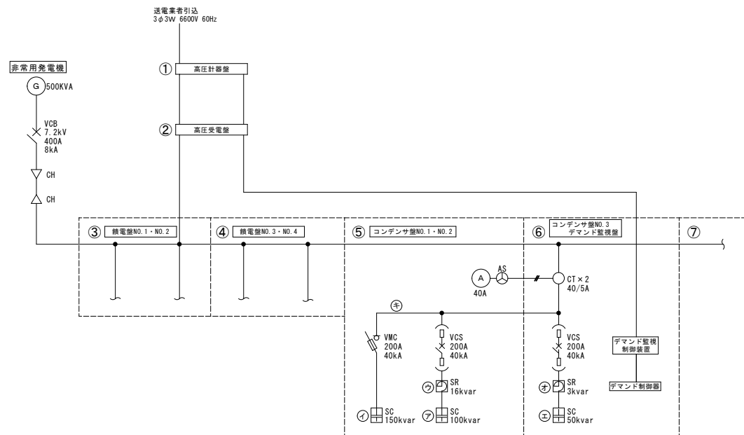
【改修前】受電所屋内キュービクル 単線結線図 S=1/X
