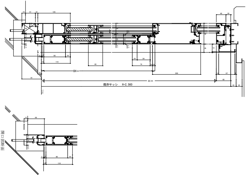
建具(ハンガードア)標準詳細図 1:X
