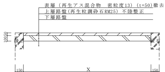
補修前標準舗装断面詳細図 S = 1 : 3 0
