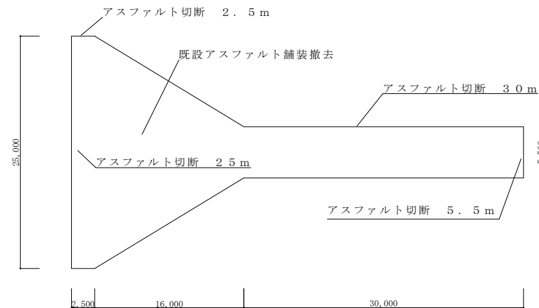
施工場所3 補修前平面図 S = 1 : 4 0 0
