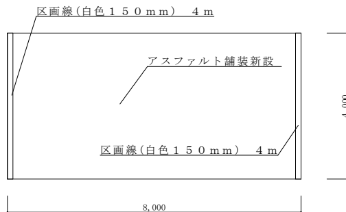
施工場所2 補修後平面図 S = 1 : 1 0 0
