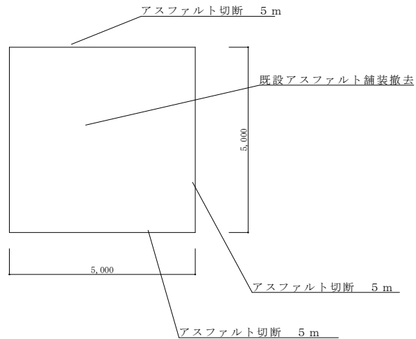
施工場所1 補修前平面図 S = 1 : 1 0 0
