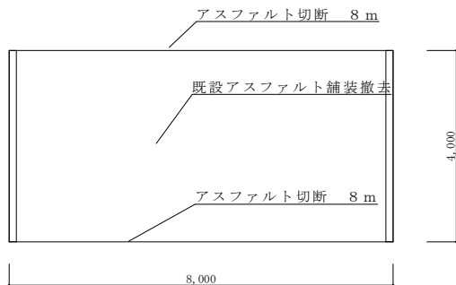
施工場所2 補修前平面図 S = 1 : 1 0 0
