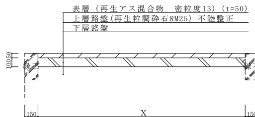
補修後標準舗装断面詳細図 S = 1 : 3 0
