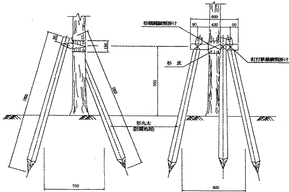
側面図
