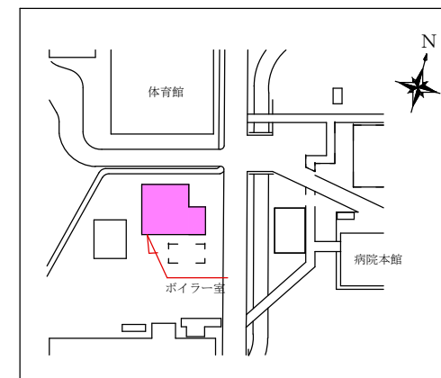
配置図 S=1:X
