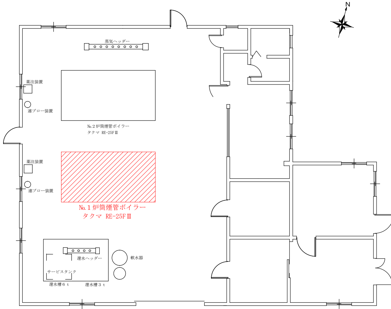
ボイラー室平面図 S=1:80
