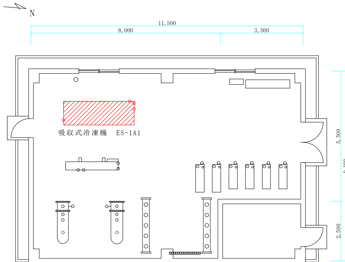
38号機械室平面図
