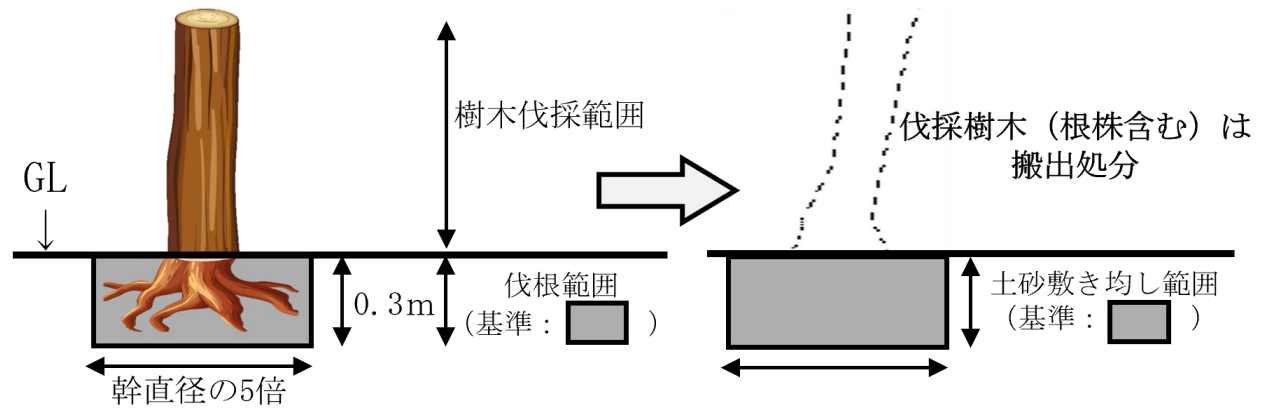
樹木伐採・伐根要領
