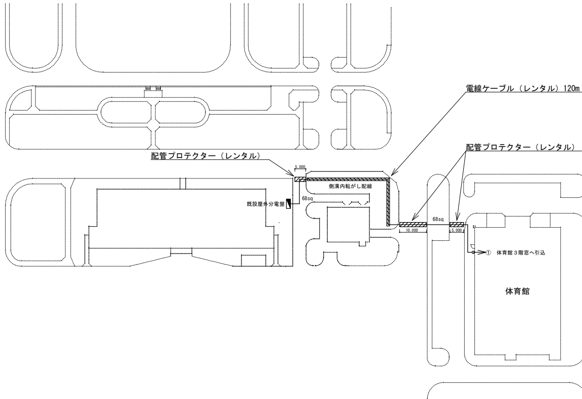
屋外配置図 1/1000
