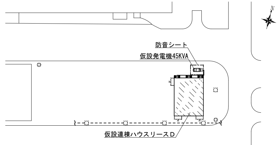
詳細配置図 S=1/500
