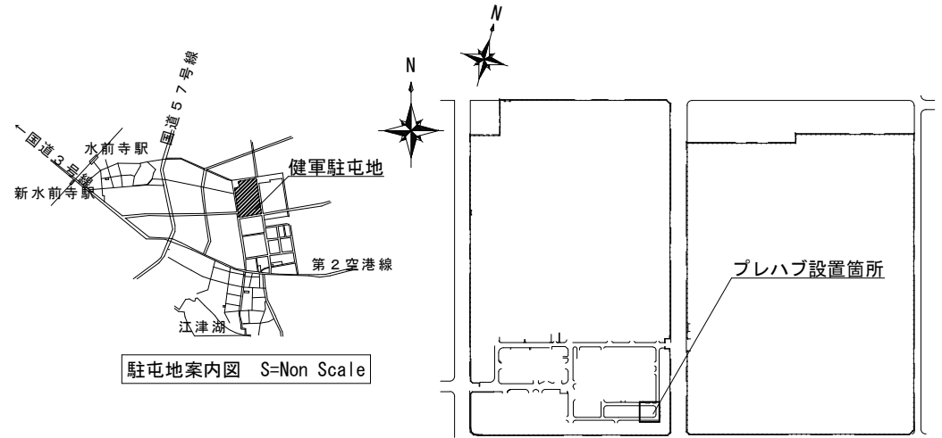
配置図 S=1:X
