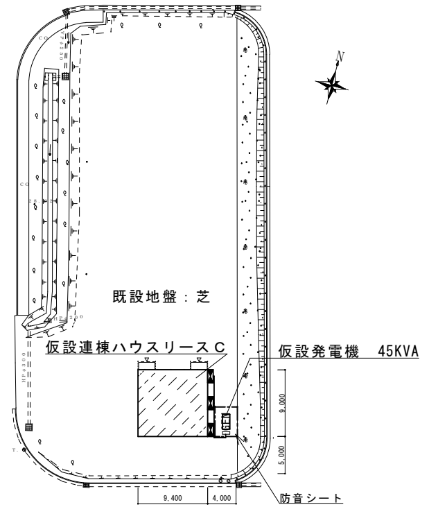
詳細配置図 S=1:500
