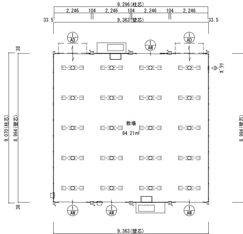
平面図 S=1:100
