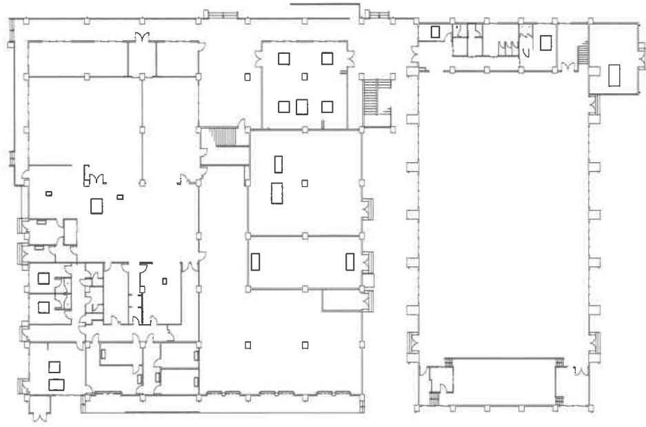
空調設備平面図 (5号1F) 1/400
