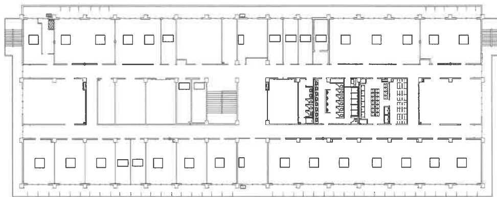
空調設備平面図 (4号2F) 1/500
