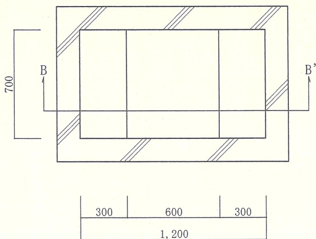
油分離槽③ 平面圖
