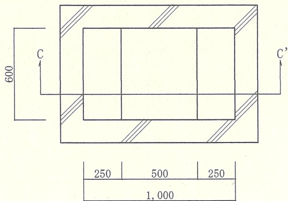
油分離槽② 平面圖
