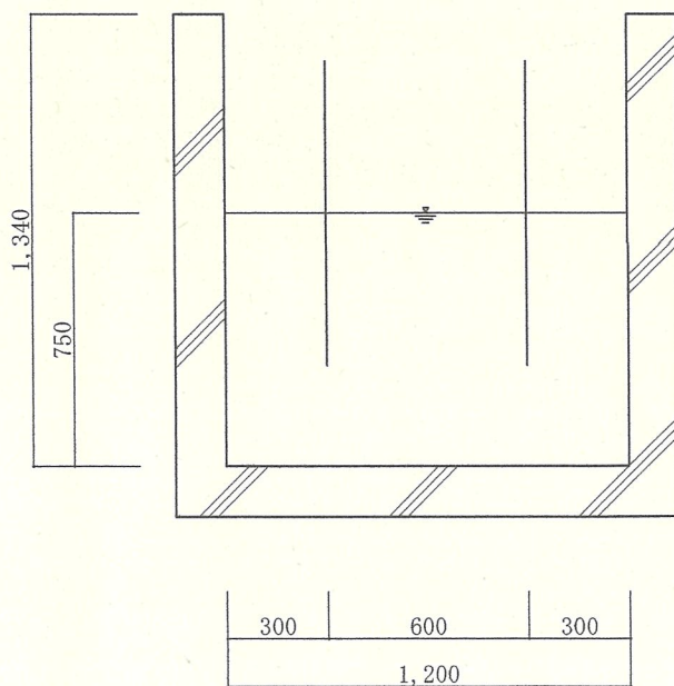
油分離槽③ B-B' 断面圖
