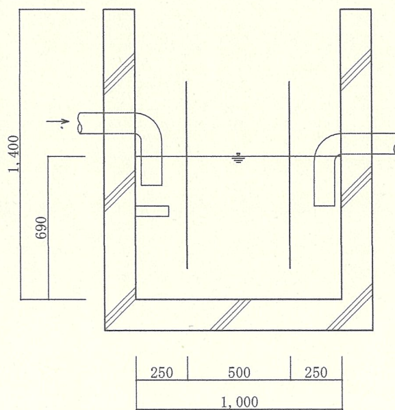
油分離槽② C-C' 断面圖
