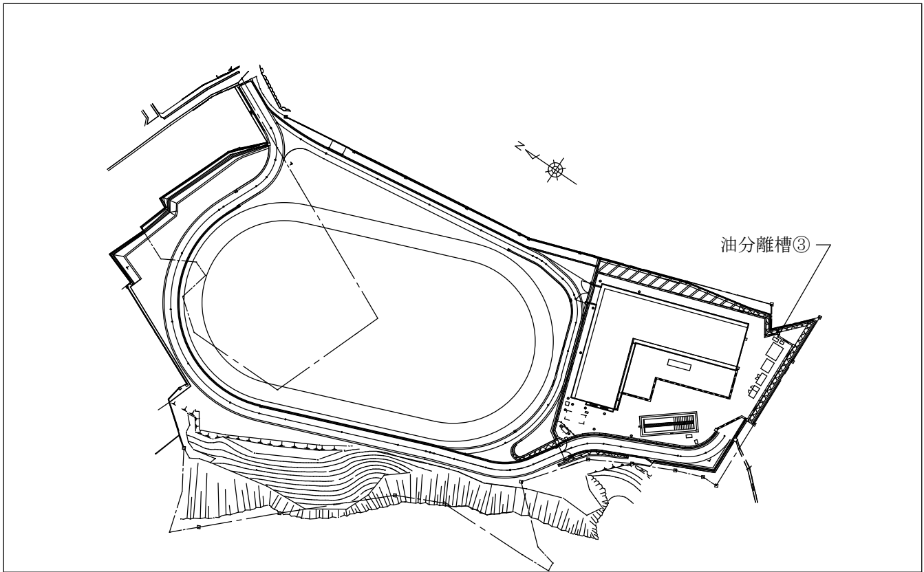
訓練場配置図 S = 1 / X
