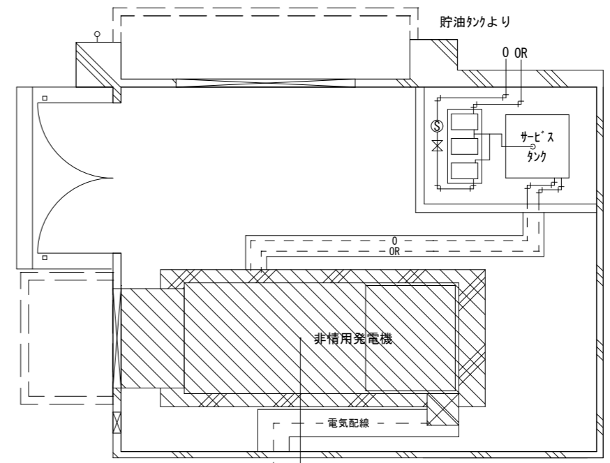
23号建物発電機室 S=1:100
