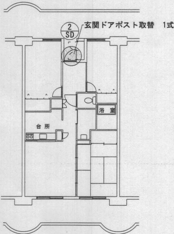
阿波根宿舎平面図 S=1:150
