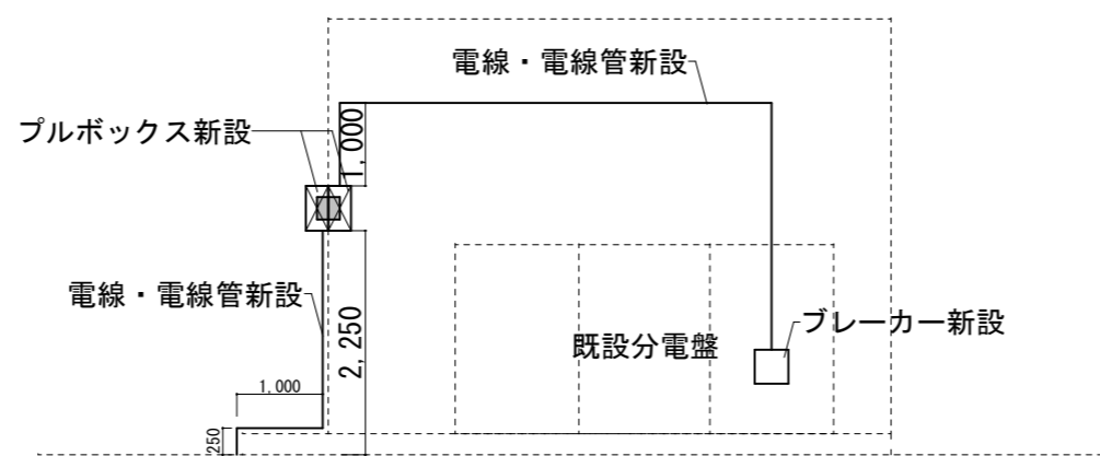
B-B'断面図 S=1/75 凡例: ■ コア抜き箇所
