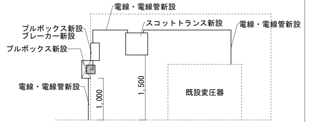
B-B'面断面図 S=1/50 凡例：■ コア抜き箇所
