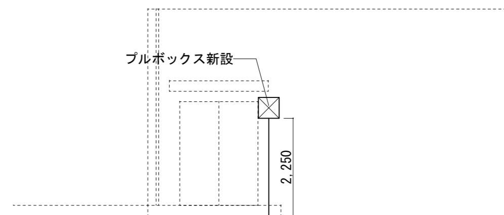
A面立面図 S=1/75
