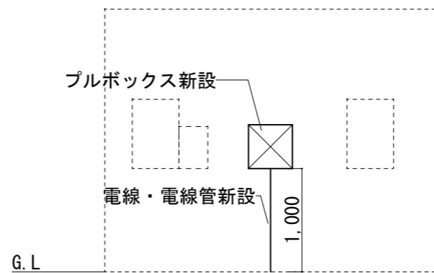
A面立面図 S=1/50
