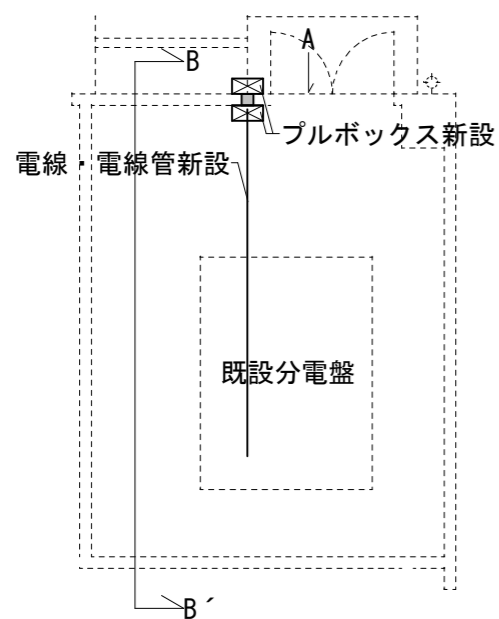
53号建物電気室平面図 S=1/50 凡例: ■ コア抜き箇所
