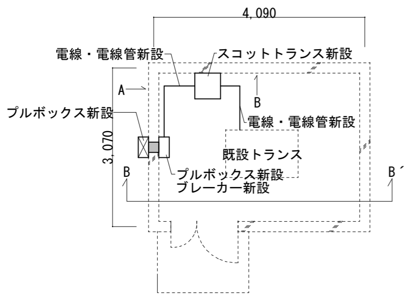
3号建物平面図 S=1/75 凡例：■ コア抜き箇所
