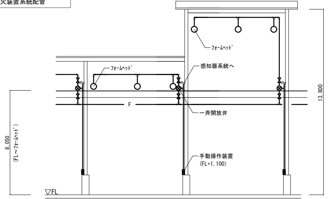
立面図 S=1/200
