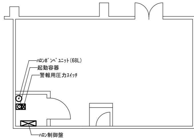
1F機械室平面図 S=1/300
