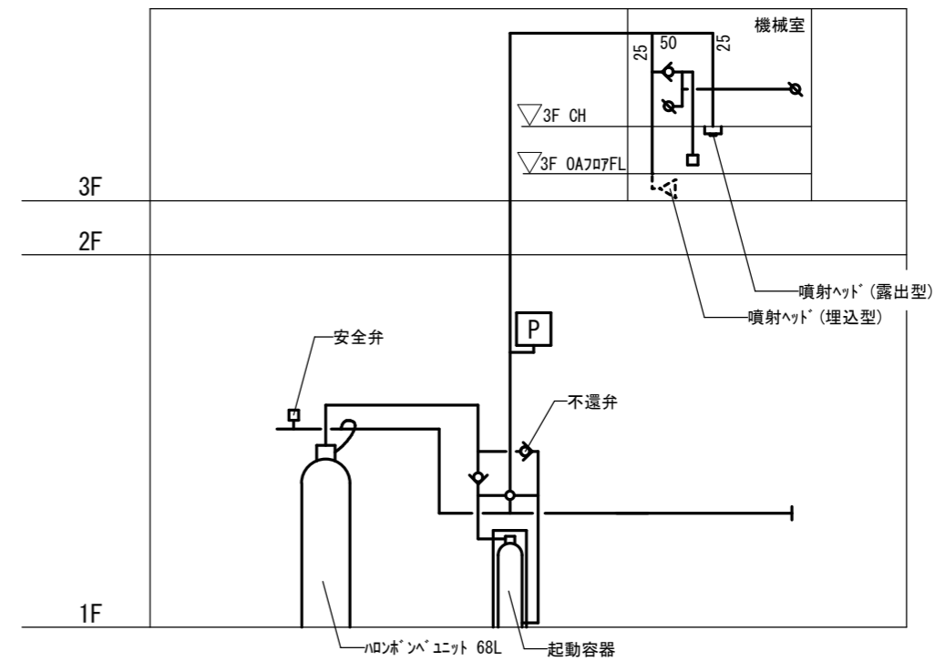
ハロン消火配管系統図 S=1/X
