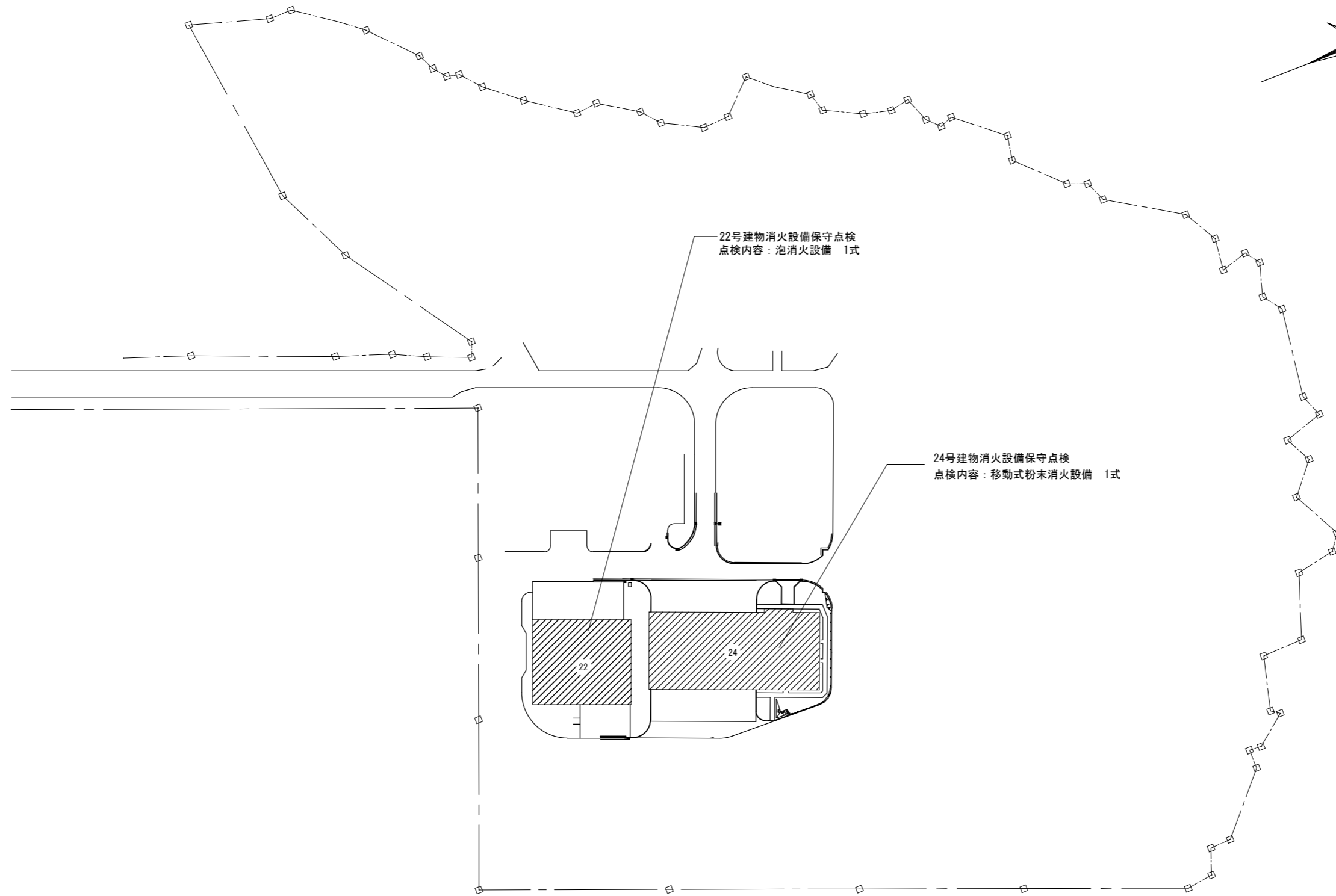
八重瀬分屯地配置図 S=1/2,000
