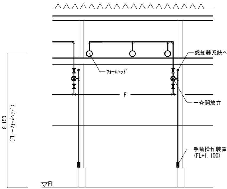
立面図 S=1/200
