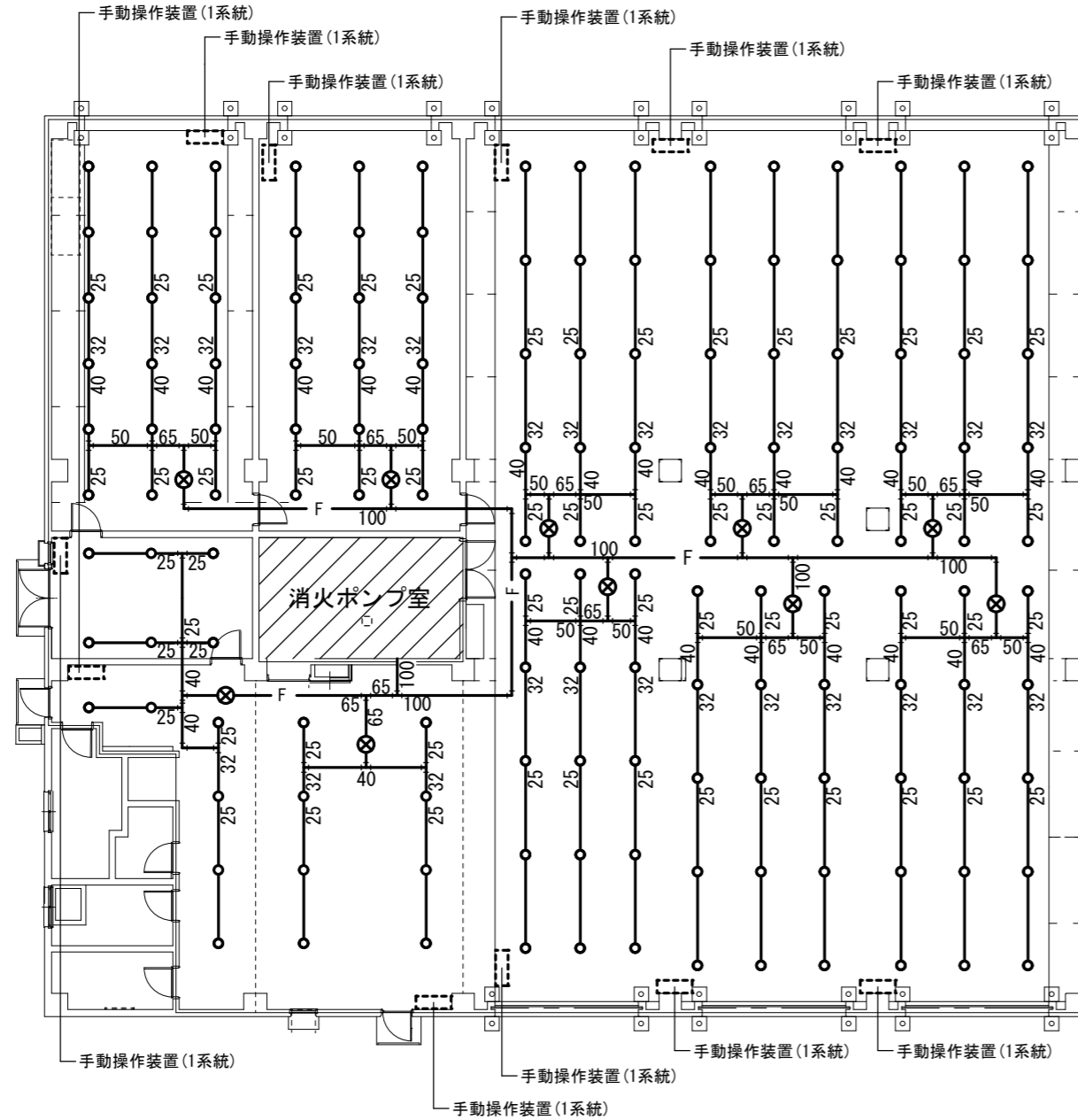
八重瀬22号建物平面図 S=1/300
