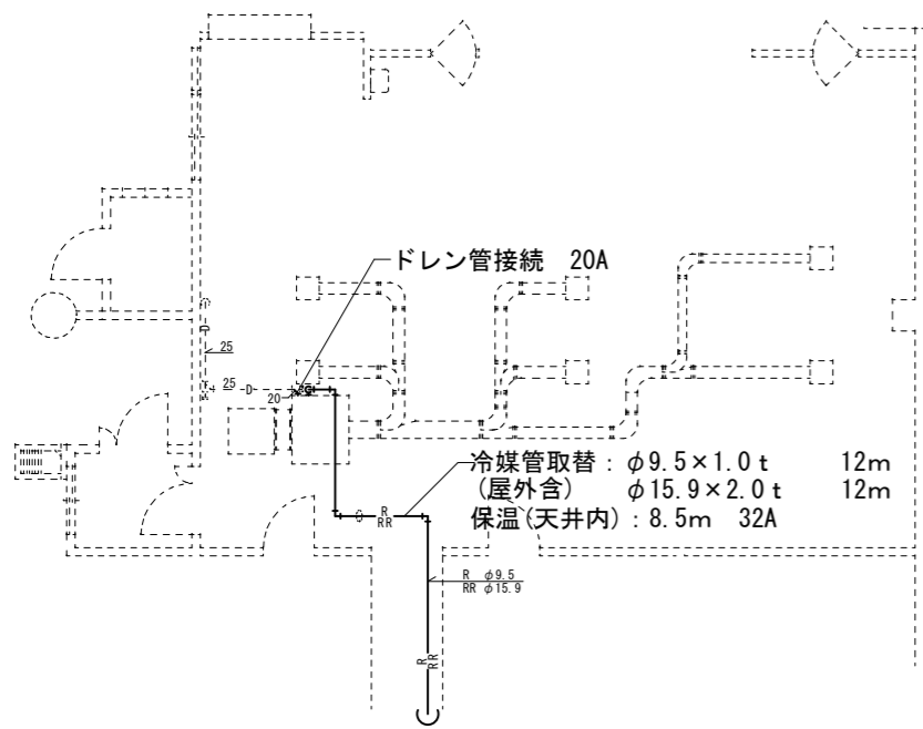
1階食堂厨房平面詳細図 S=1/150
