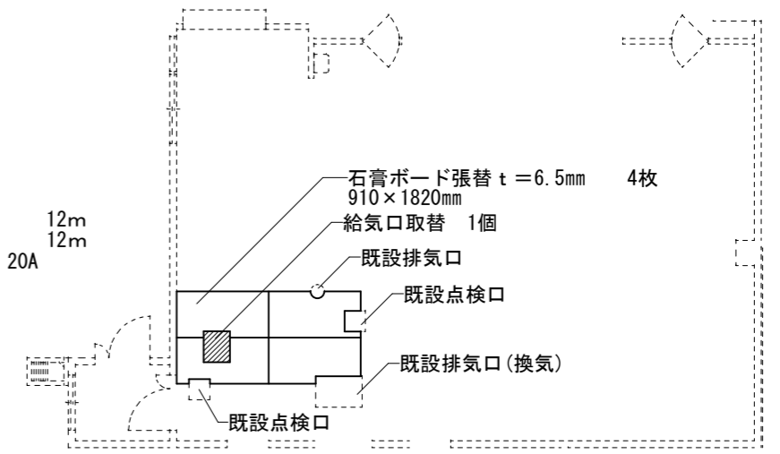
1階食堂厨房天井伏図 S=1/150
