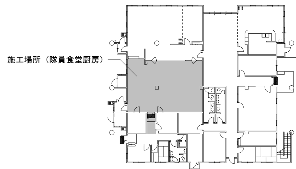
12号建物平面図 S=1/400
