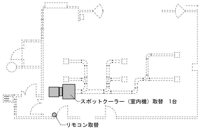
1階食堂厨房平面詳細図 S=1/150
