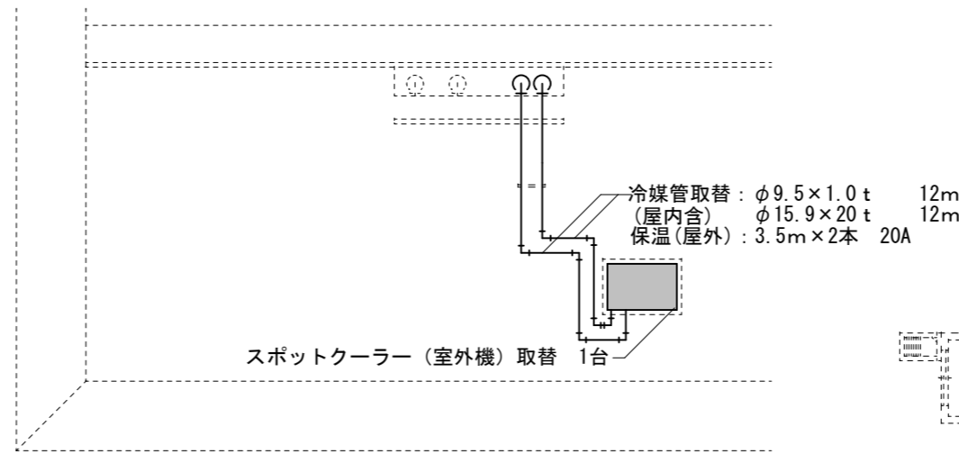
RF階平面詳細図 S=1/150
