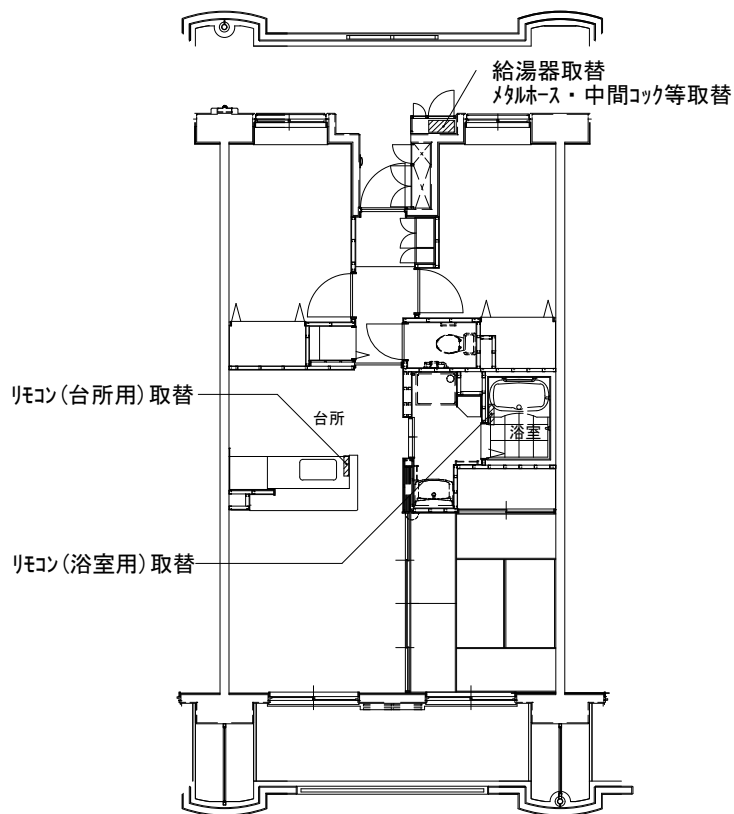
賀数宿舎5号棟平面図 S=1:150
