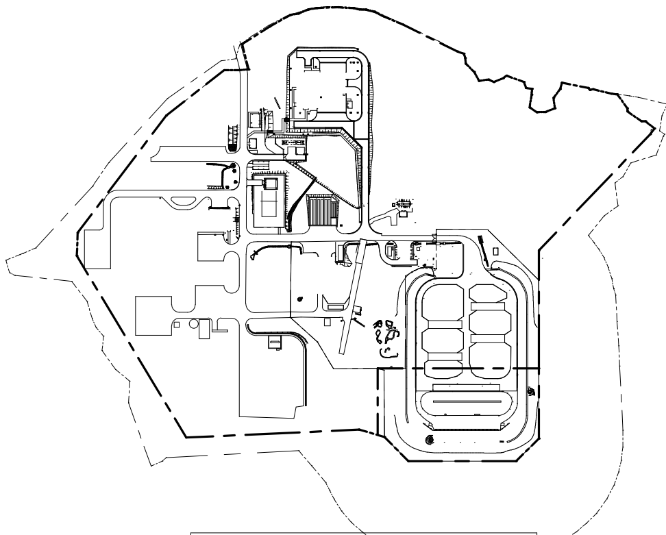
知念分屯地配置図 S=1/4000
