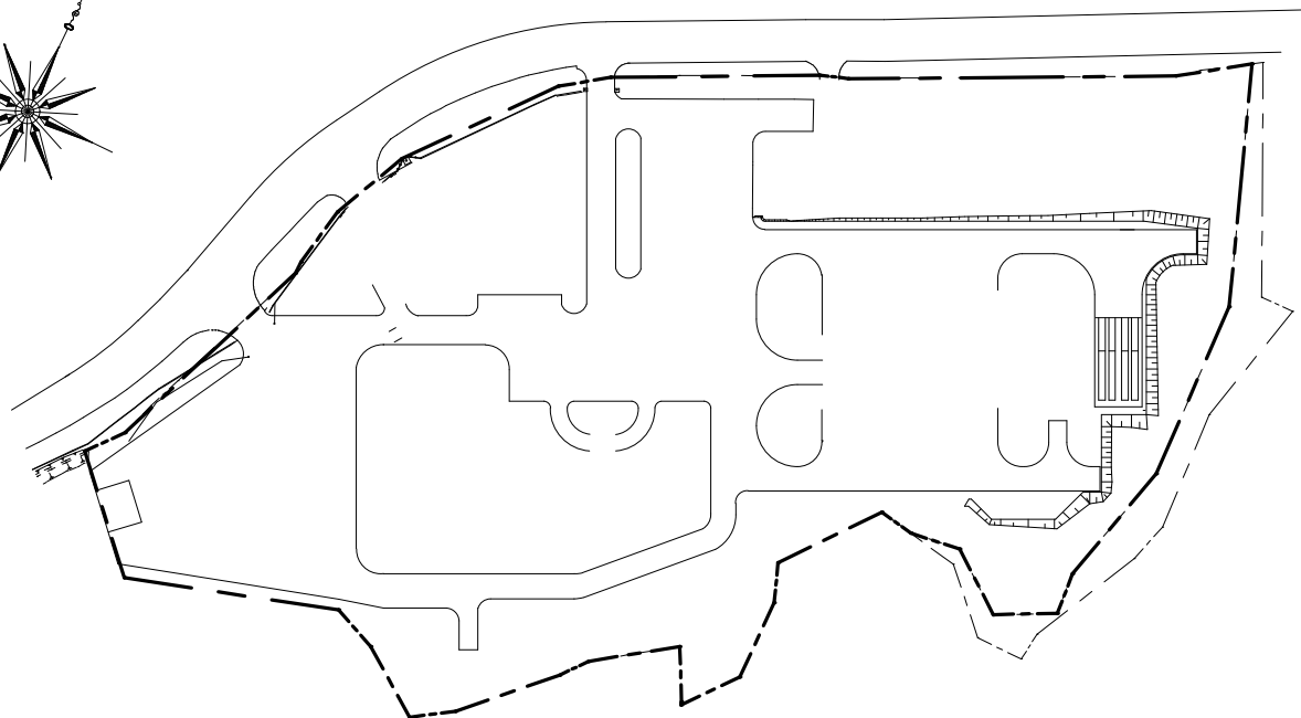
白川分屯地配置図 S=1/2000
