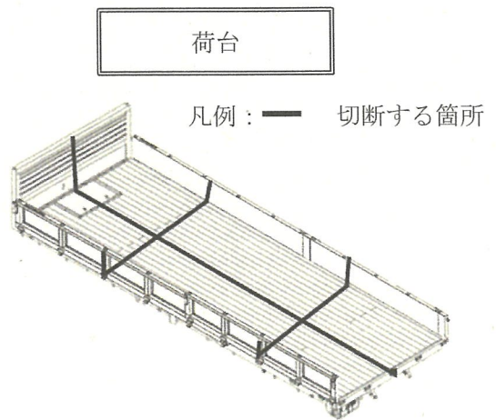
図5-特大型トラック外装部品及びフレームの解体図
