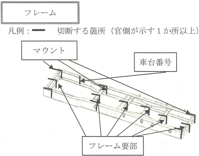
図5-特大型トラック外装部品及びフレームの解体図
