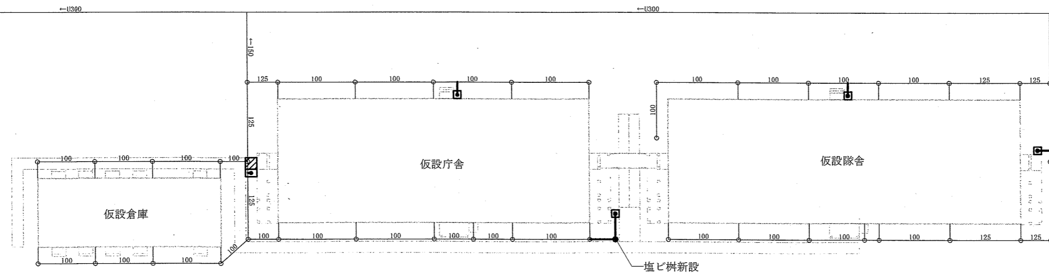
雨水排水設備平面図 (1/500)
