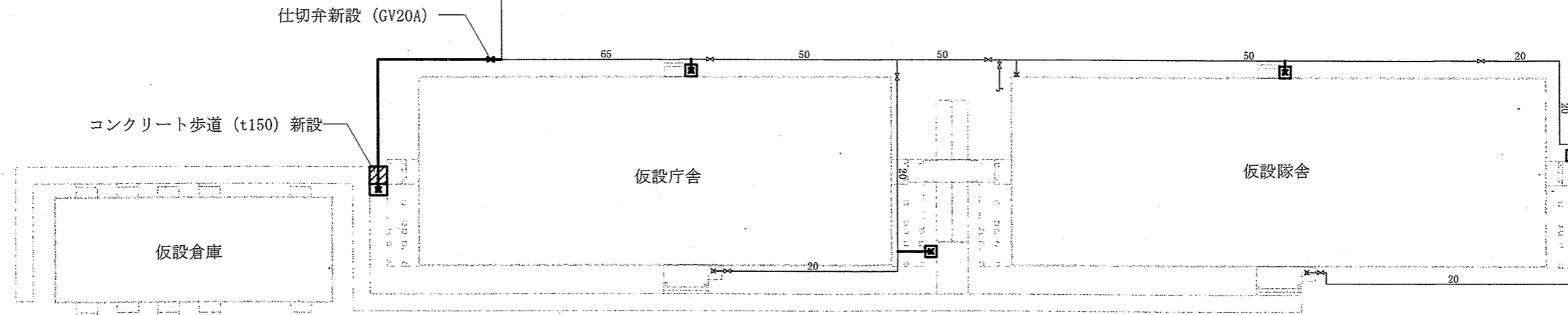
給水設備平面図 (1/500)
