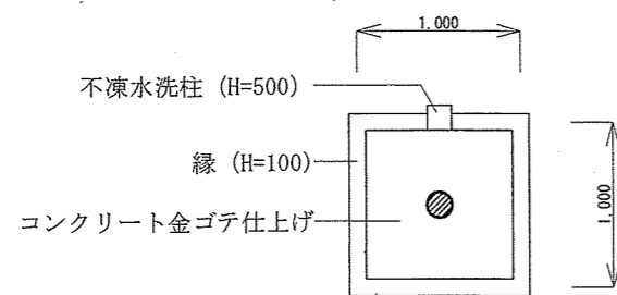
靴洗い場標準図 (1/50)
