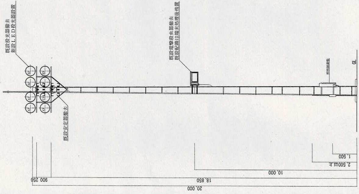
照明柱立面図 S = 1:100
