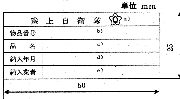
図1-銘板
