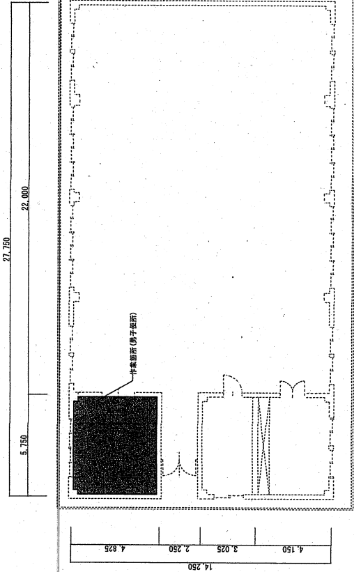
561号建物1階平面図 1/200
