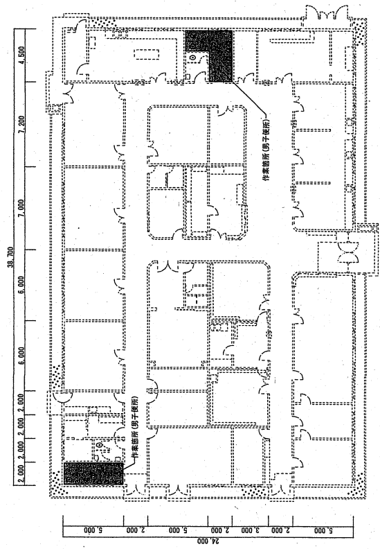
590号建物1階平面図 1/300
