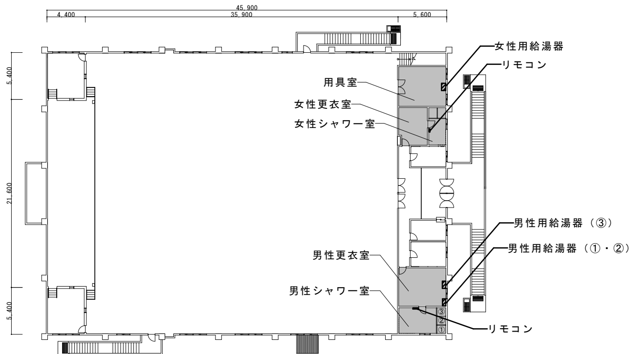
体育館 2階平面図
