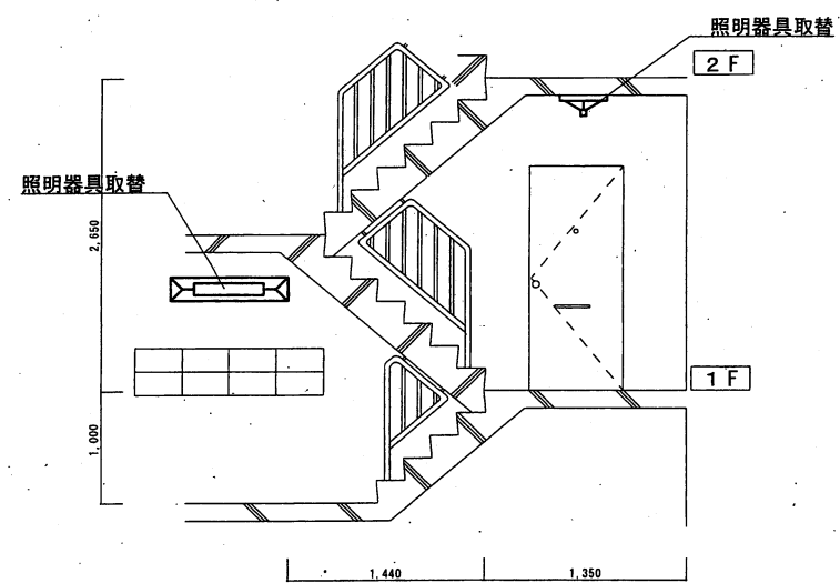
七福宿舍階段部立面図 S=1/X
