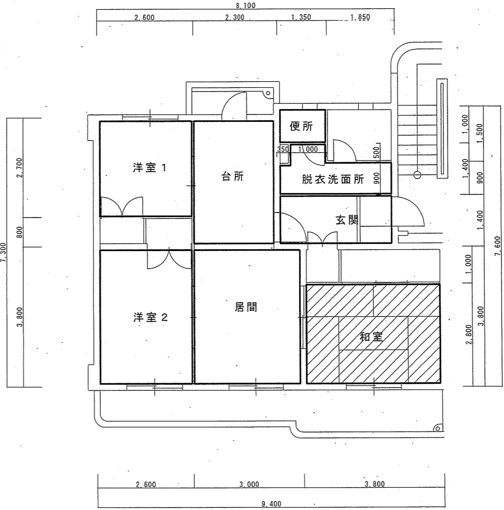
宿舎平面図 S=1/100
