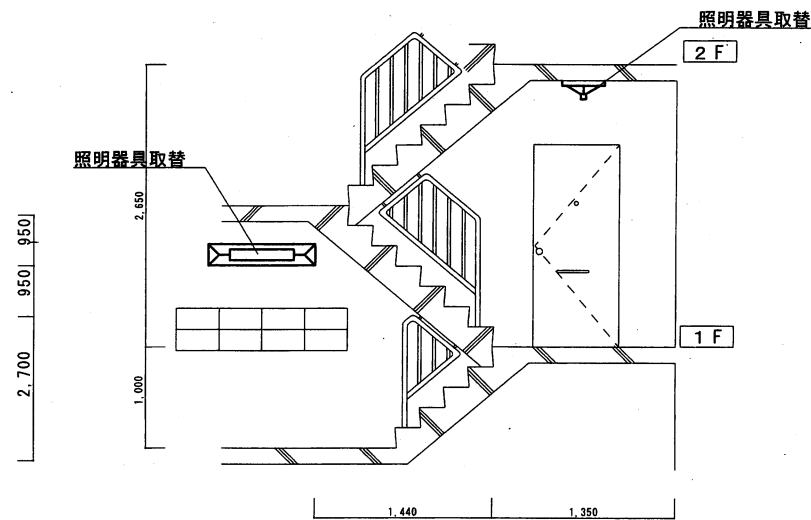
七福宿舍階段部立面図 S=1/X
