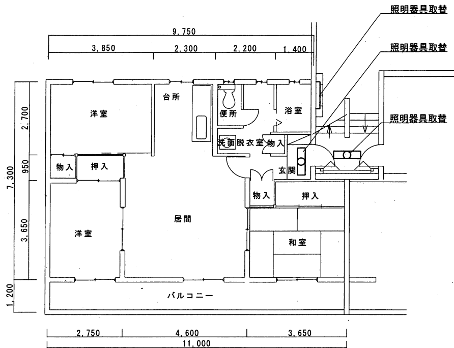
七福宿舍平面図 S=1/100
