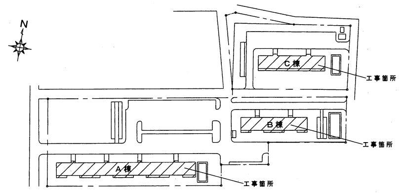
七福宿舍配置図 S=1/1500
